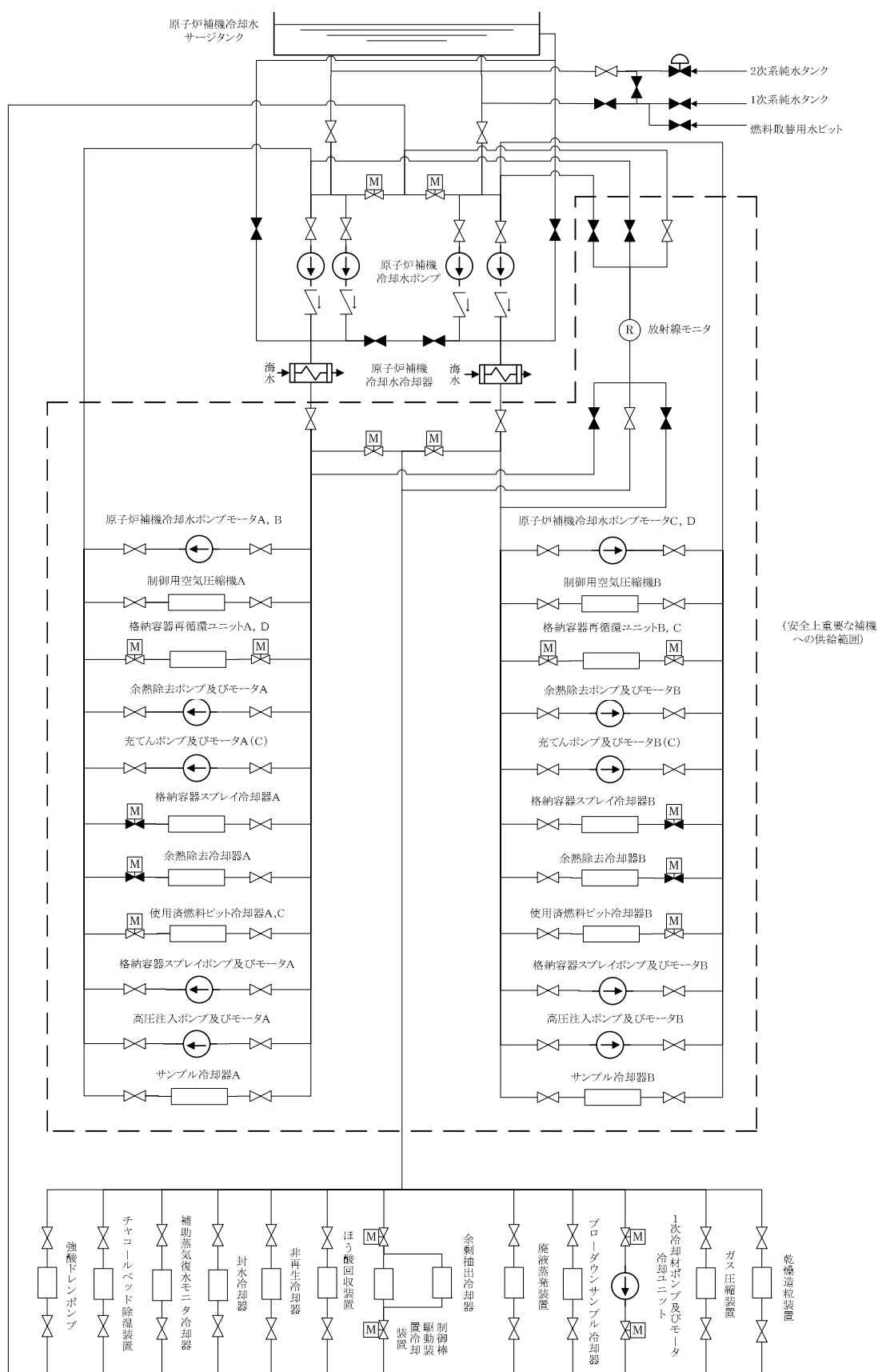
大飯発電所 4 号機の系統構成 (原子炉補機冷却水系)
