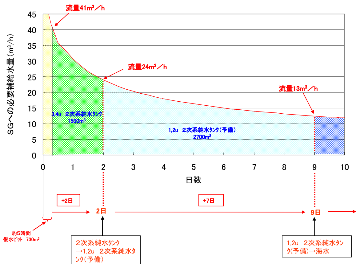
図3. 補給水量と水源
