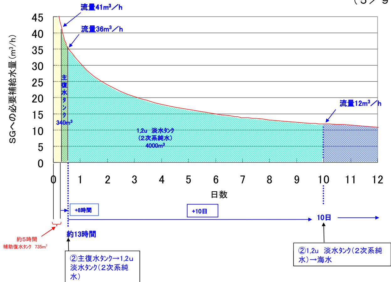
図 4 補給水量と水源 (シナリオ 2 : 主復水タンク→1, 2u 淡水タンク)
