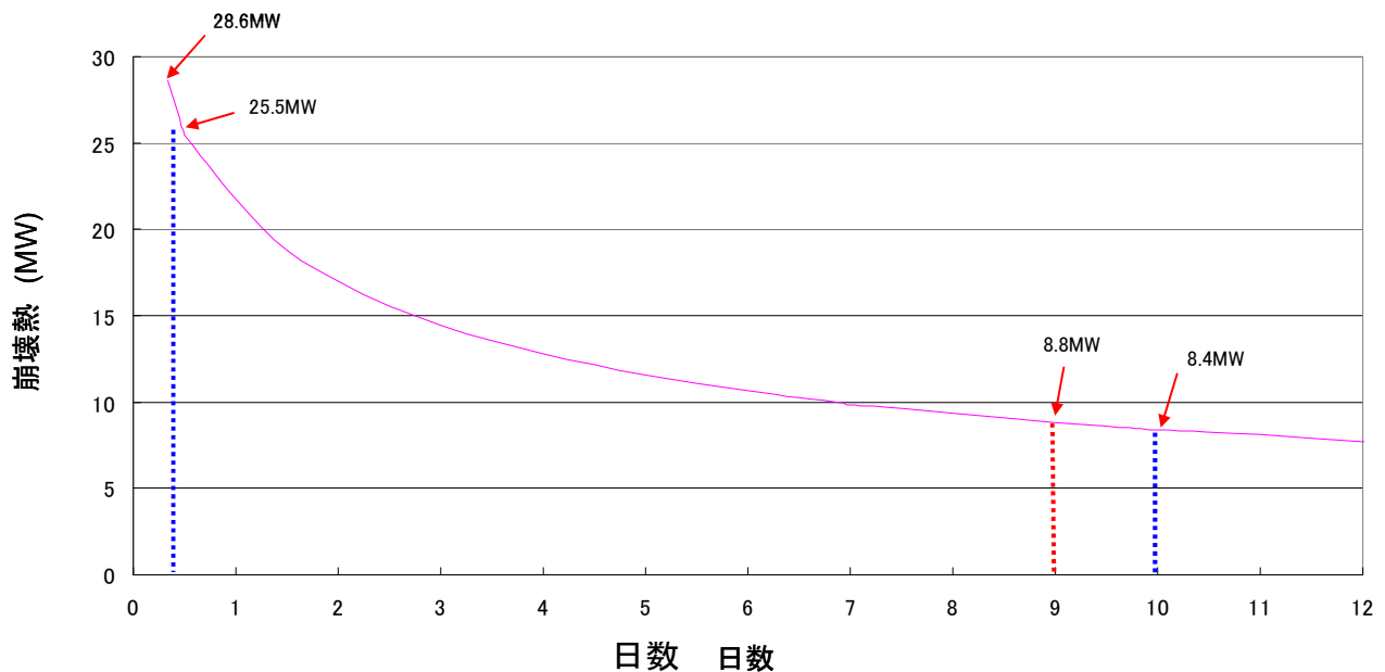
図2. 崩壊熱の変化
