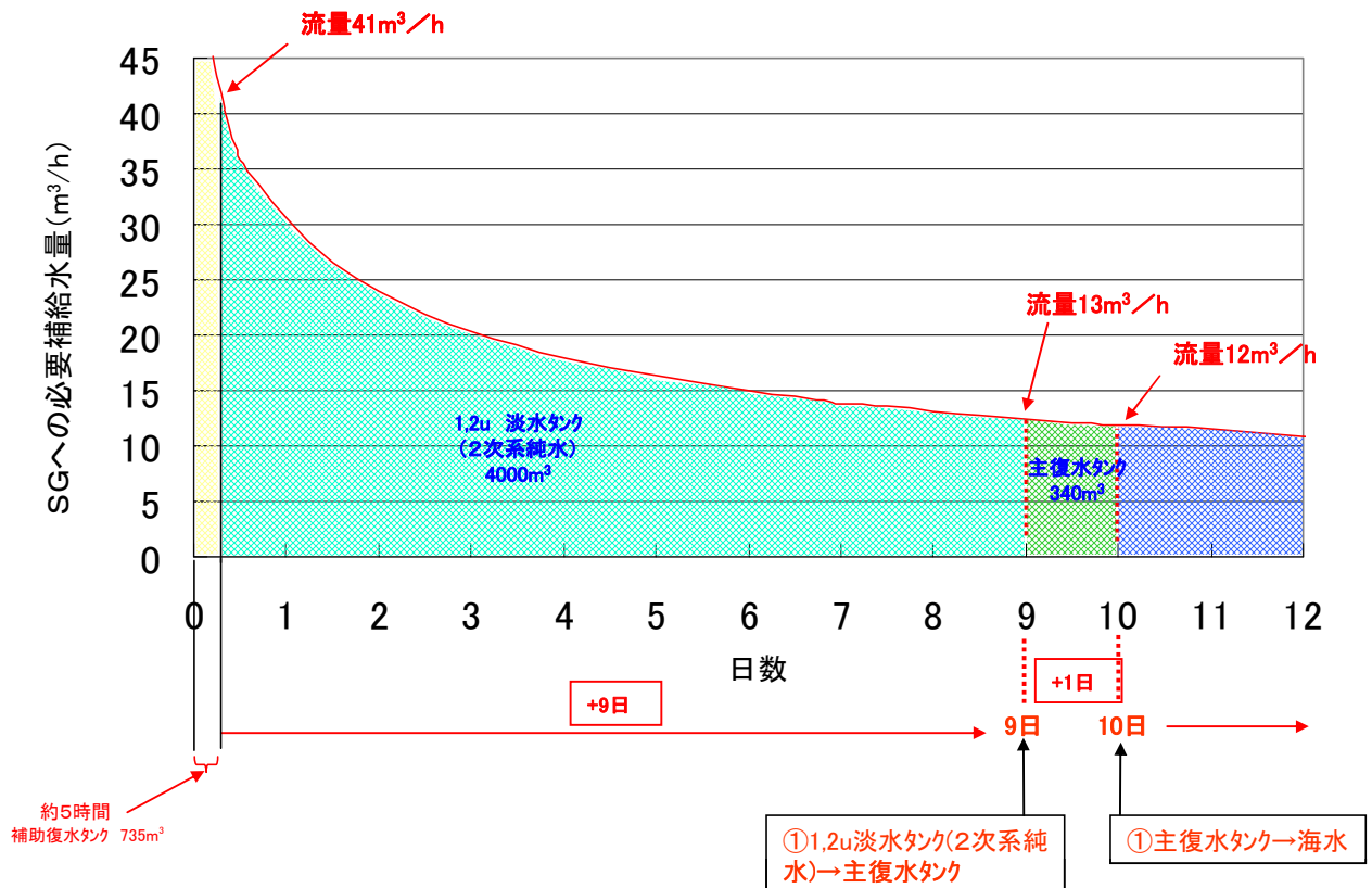
図3 補給水量と水源 (シナリオ 1 : 1,2u 淡水タンク→主復水タンク)
