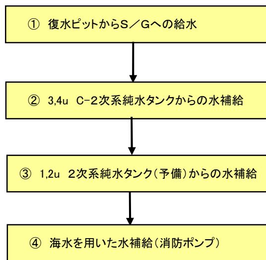
図1. 給水シナリオ
