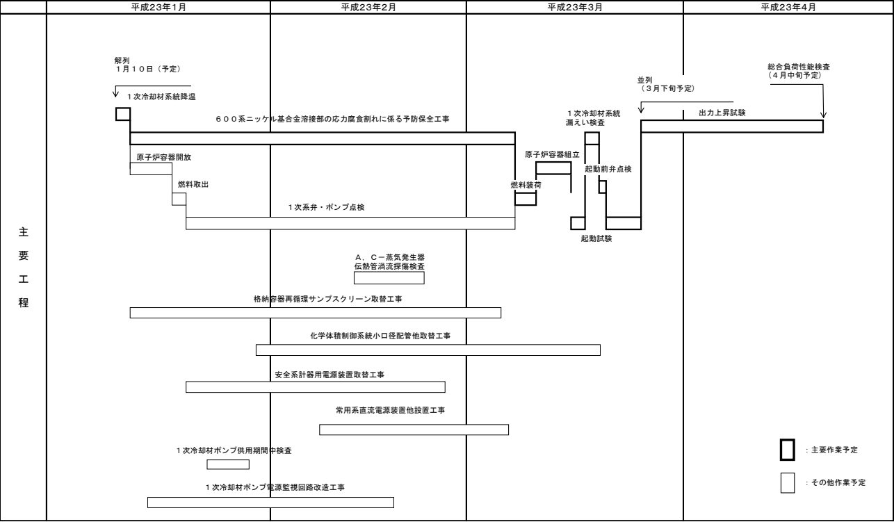
高浜発電所1号機 第27回定期検査工程表
