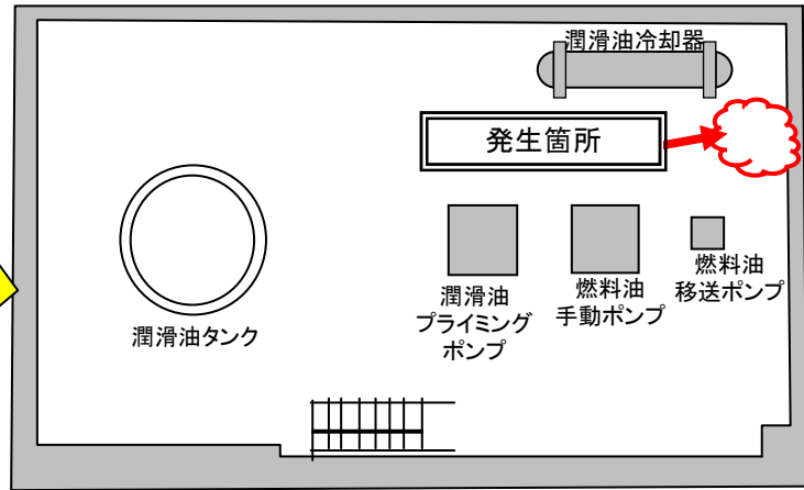
3Aディーゼル発電機室地下 平面概要図
