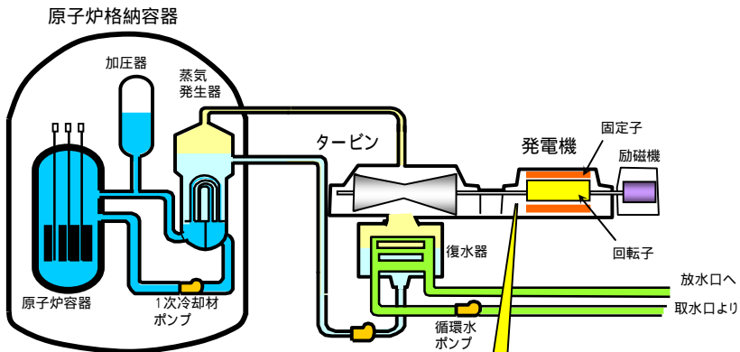
水素ガス冷却器冷却水系統概要図
