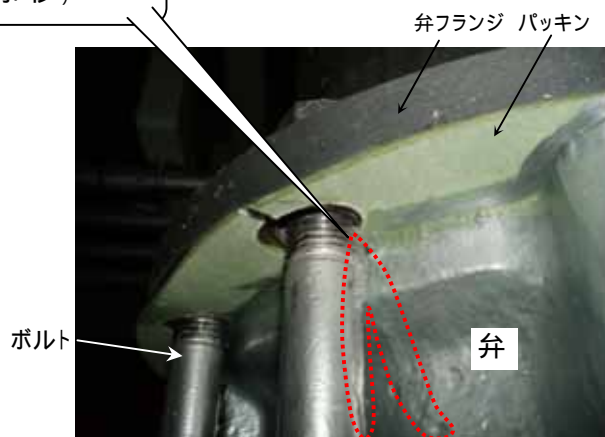
漏れ箇所の写真
