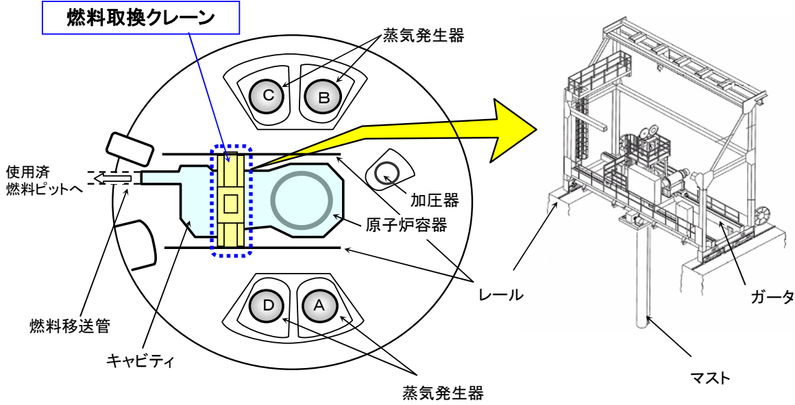
燃料取換クレーン鳥瞰図
