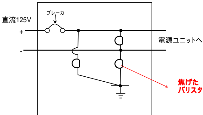
【保護回路(ブレーカ)図】
