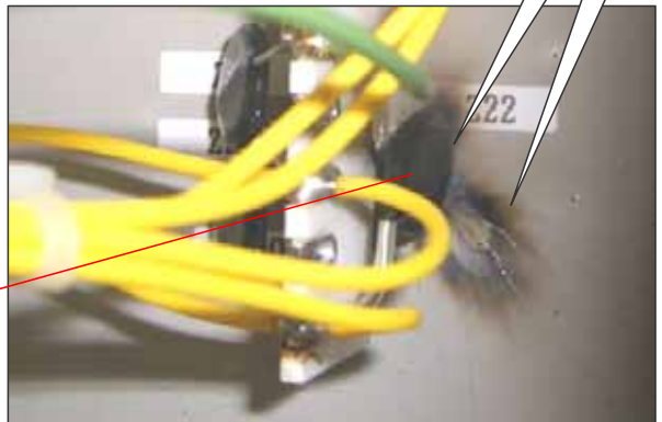
【保護回路写真】
