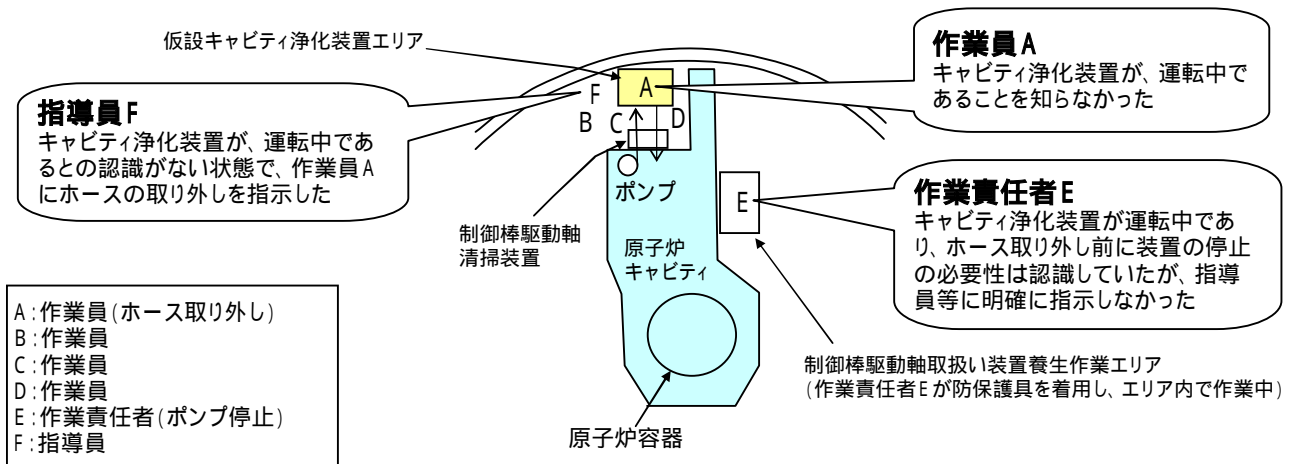
原子炉容器炉内構造物点検清掃工事作業人員配置図 (3.2mフロア)
