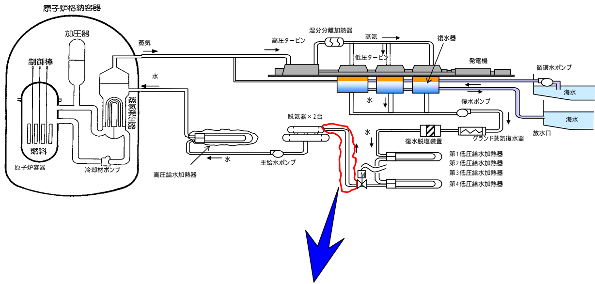
系統概略図
