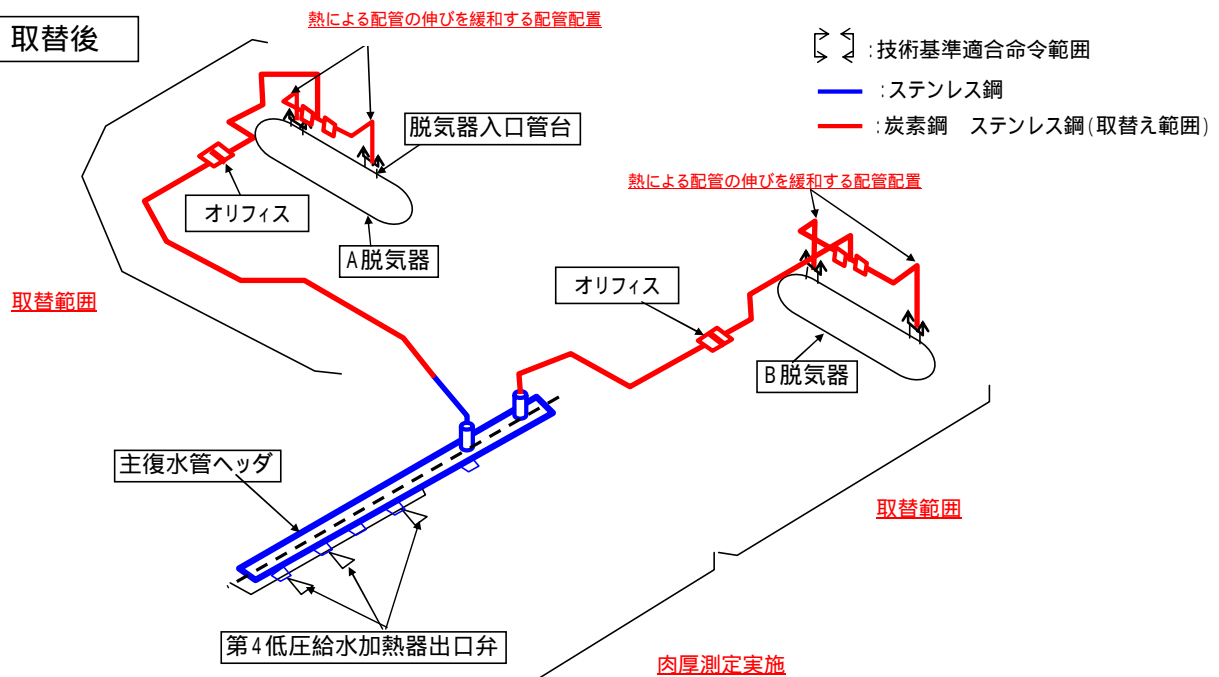
主復水ヘッダー出口～脱気器入口(今回取替範囲)の仕様比較
