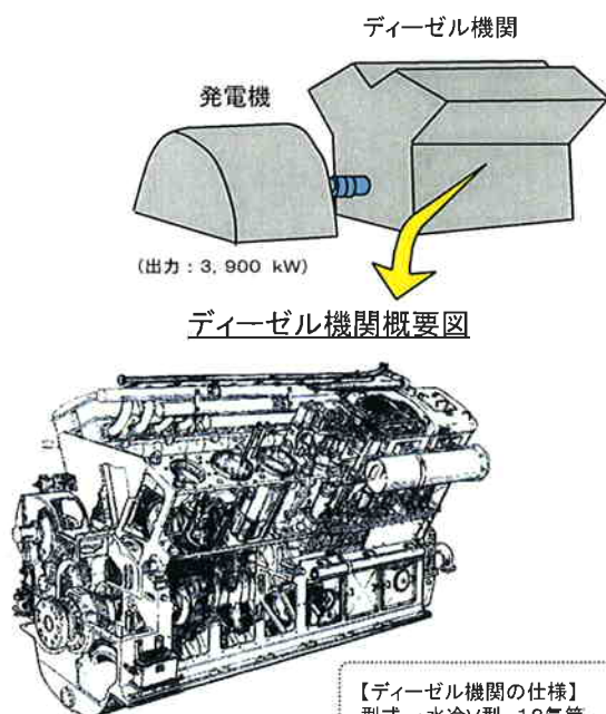
非常用ディーゼル発電機概要図
