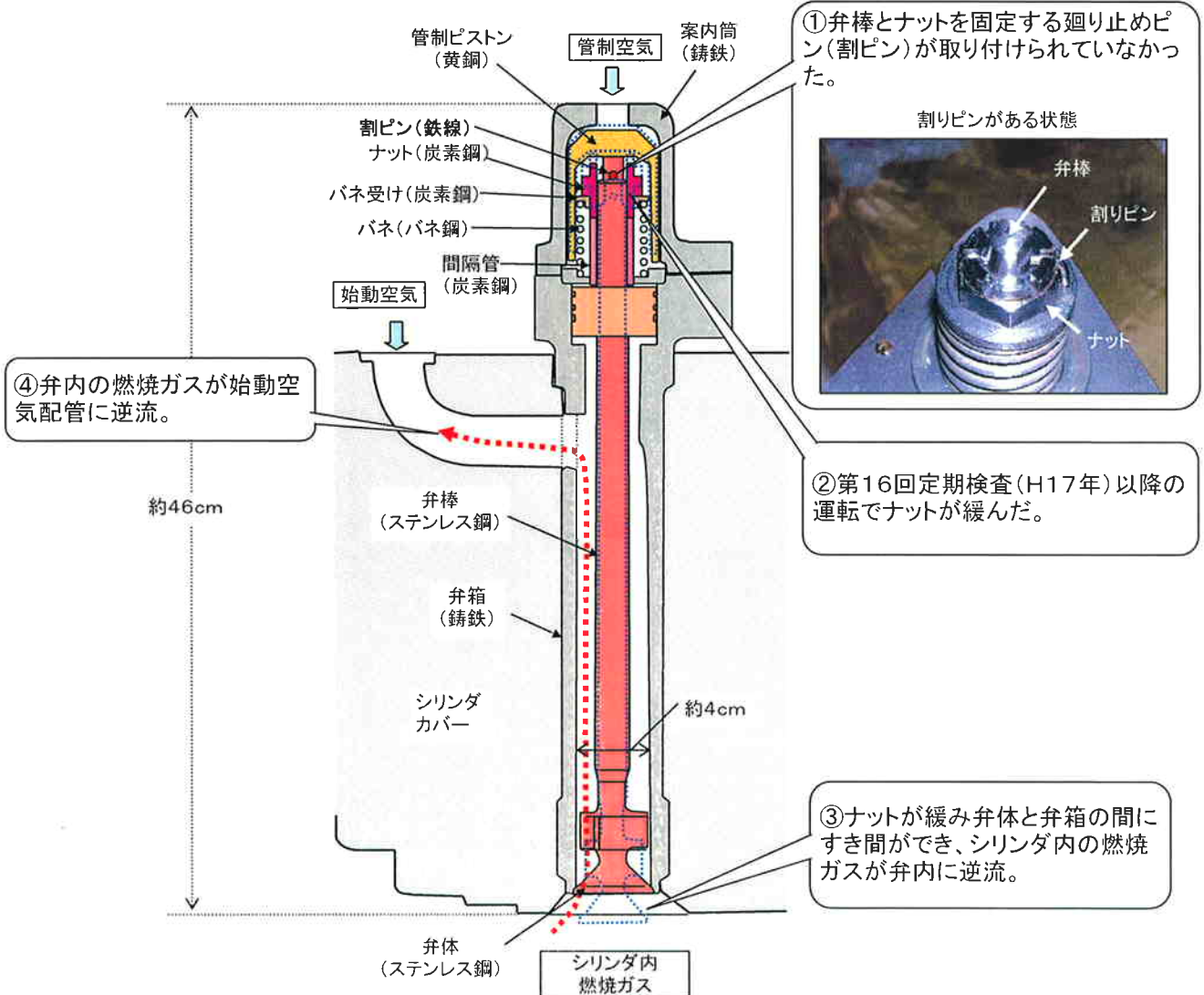
始動弁断面概要図
