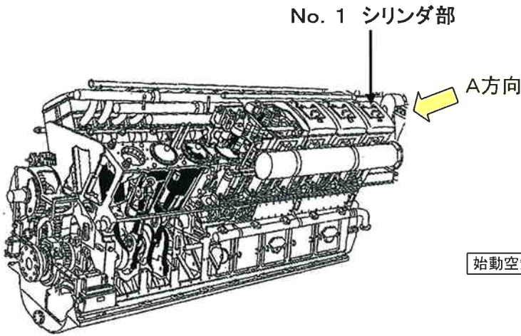
A-非常用ディーゼル発電機概要図
