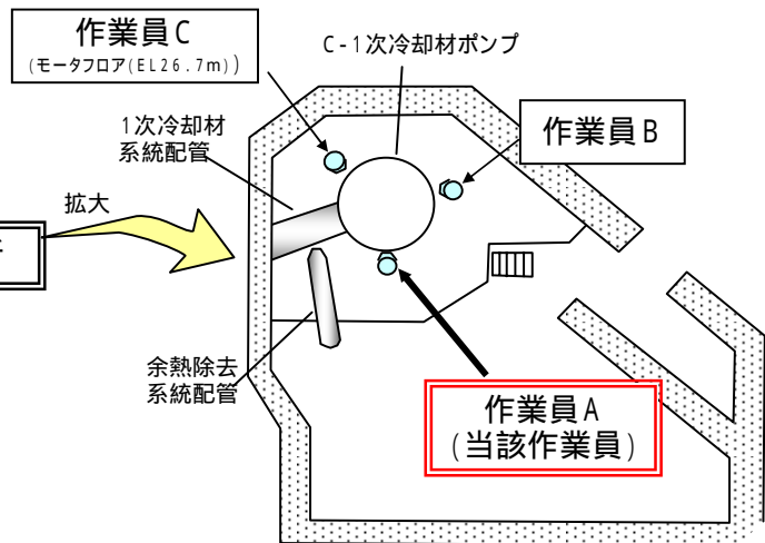
Cループ室平面概要図 (ポンプフロア(EL24.2m))
