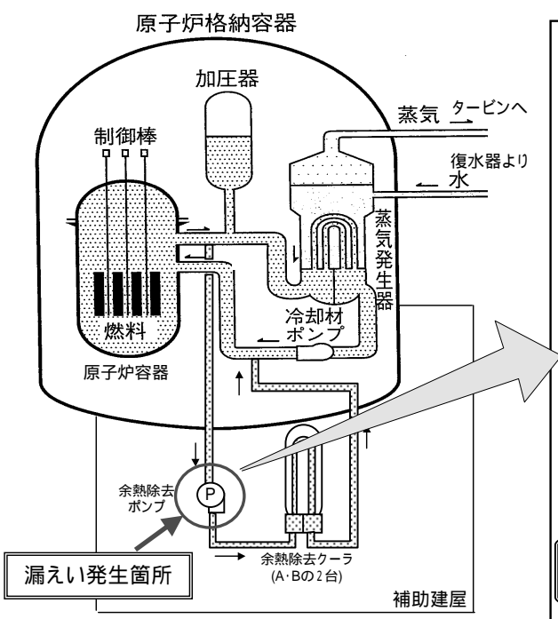
図 - 5 美浜発電所1号機 A - 余熱除去ポンプメカニカルシールからの漏えいに伴う取り替え作業(待機除外)の実施について
