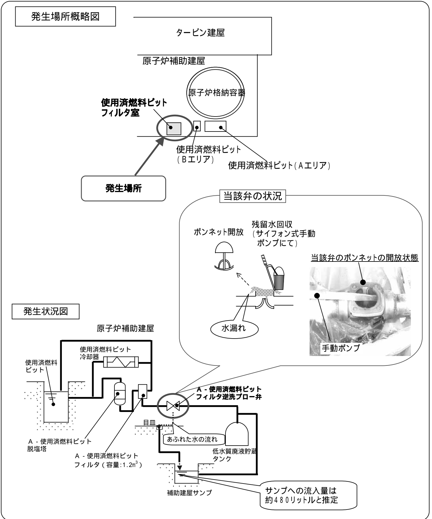
図 - 4 高浜発電所3号機 原子炉補助建屋内(管理区域内)における水漏れについて
