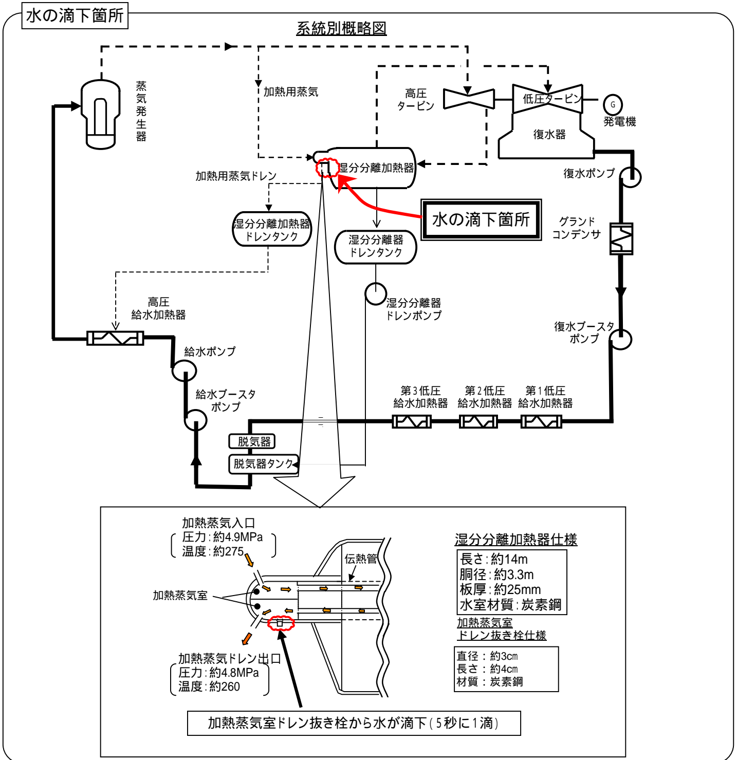
図 - 1 美浜発電所1号機 湿分分離加熱器加熱蒸気室ドレン抜き栓からの漏えいに伴う対策実施結果
