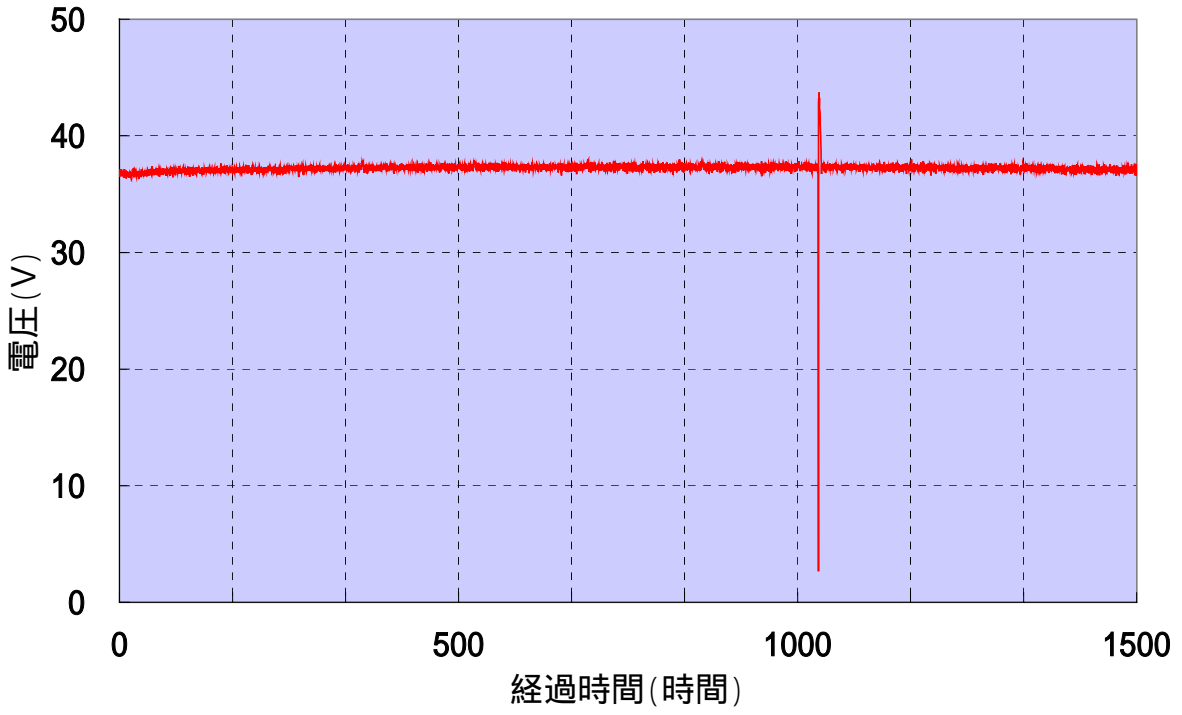
1 kW級発電システム電圧推移
