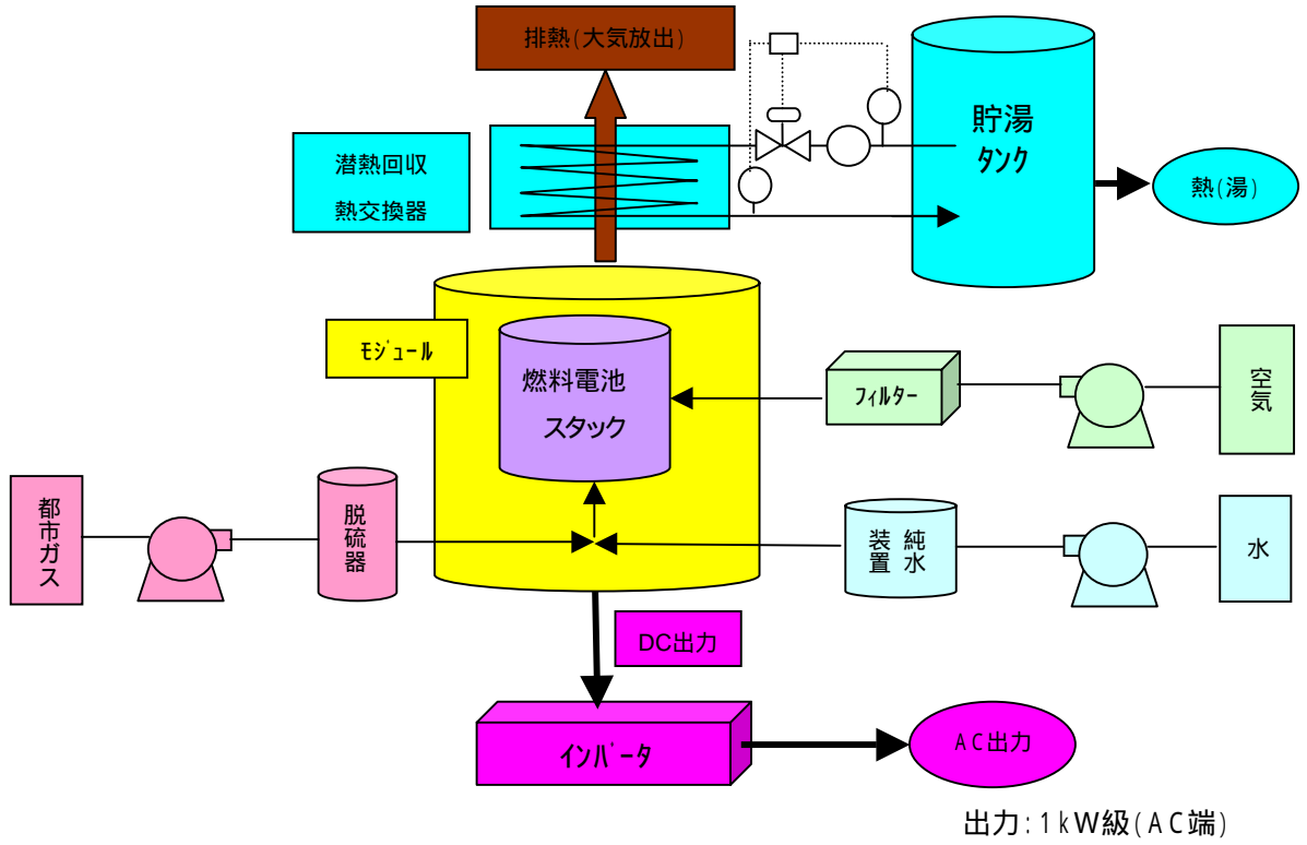
1 kW級発電システムの概念図
