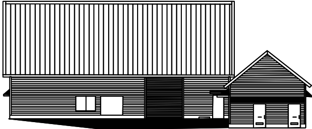
立面図
