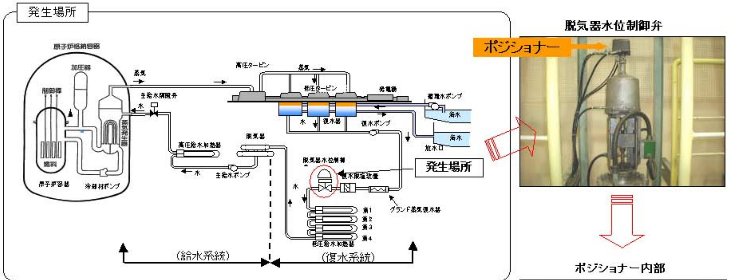
図-3 高浜発電所2号機 脱気器水位制御弁の不調について
