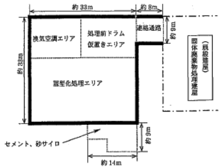
固体廃棄物固型化处理建屋平面図（2階）
