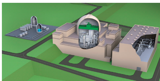
革新軽水炉(SRZ-1200)
