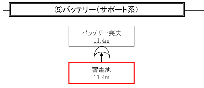
各影響緩和機能のフォールトツリー(津波:SFP燃料損傷)
