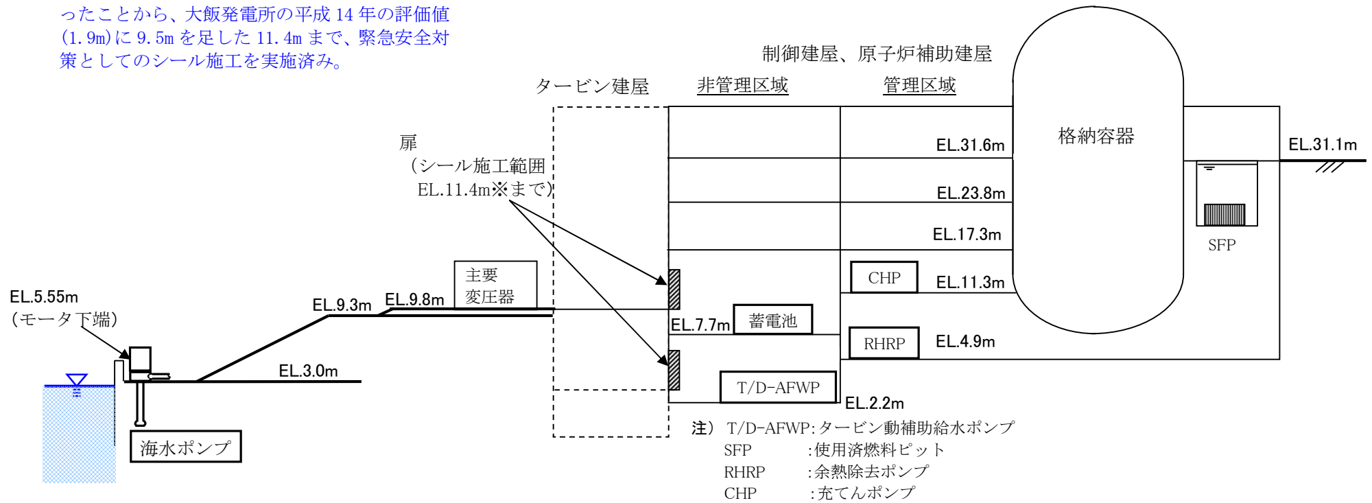
大飯1号機の敷地レベルと主要な機器等の配置レベル
