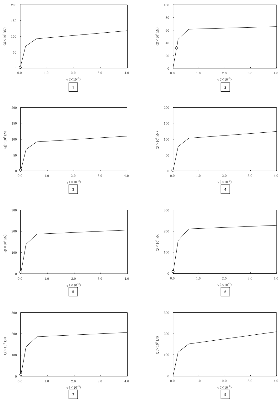
図 2-5-10 Q- \gamma 関係と最大応答値 (原子炉補助建屋 S_{S-1} NS 方向)
