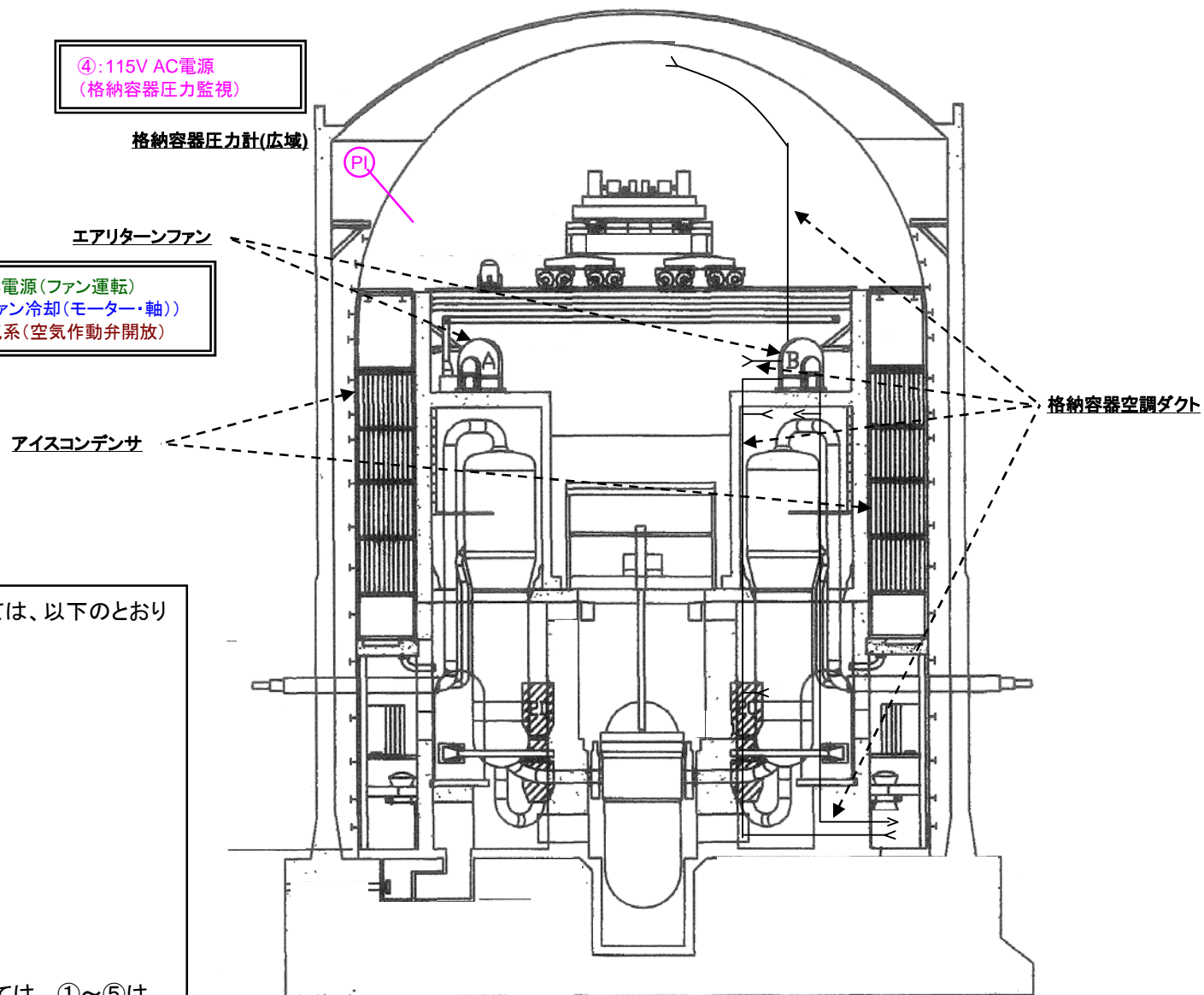
各影響緩和機能の系統図(地震: 炉心損傷)
