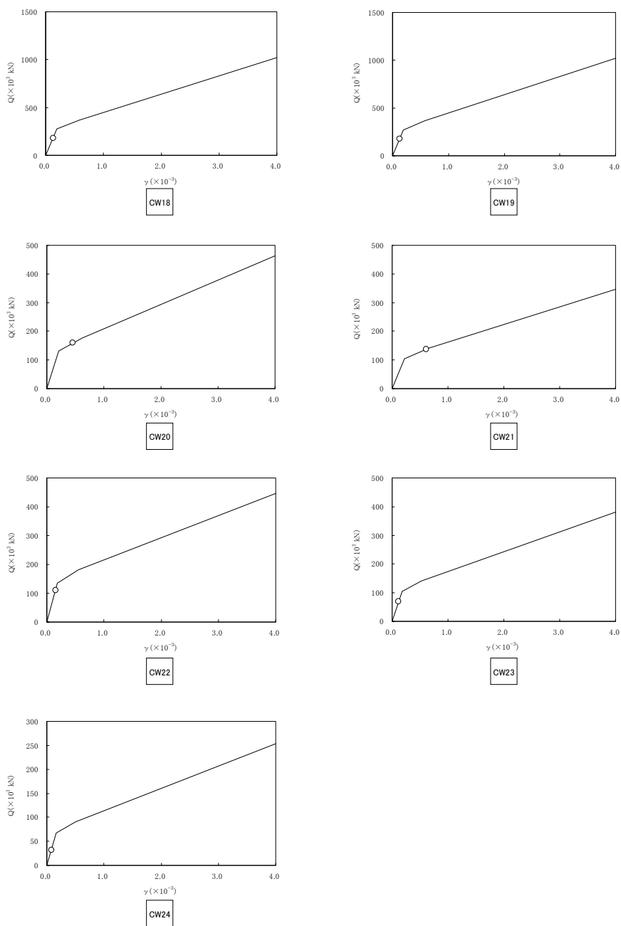
図 2-5-2 Q- \gamma 関係と最大応答値 (原子炉建屋 C/W S S-1 EW 方向)
