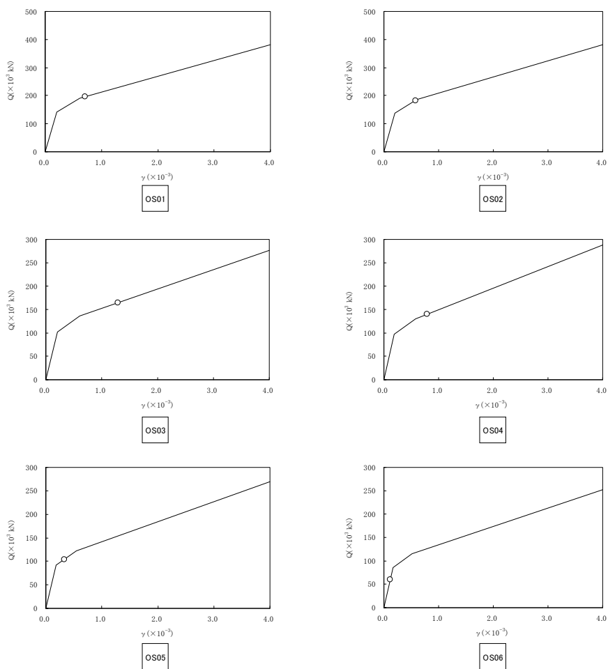
図 2-5-4 Q- \gamma 関係と最大応答値 (原子炉建屋 0/S S S-1 NS 方向)
