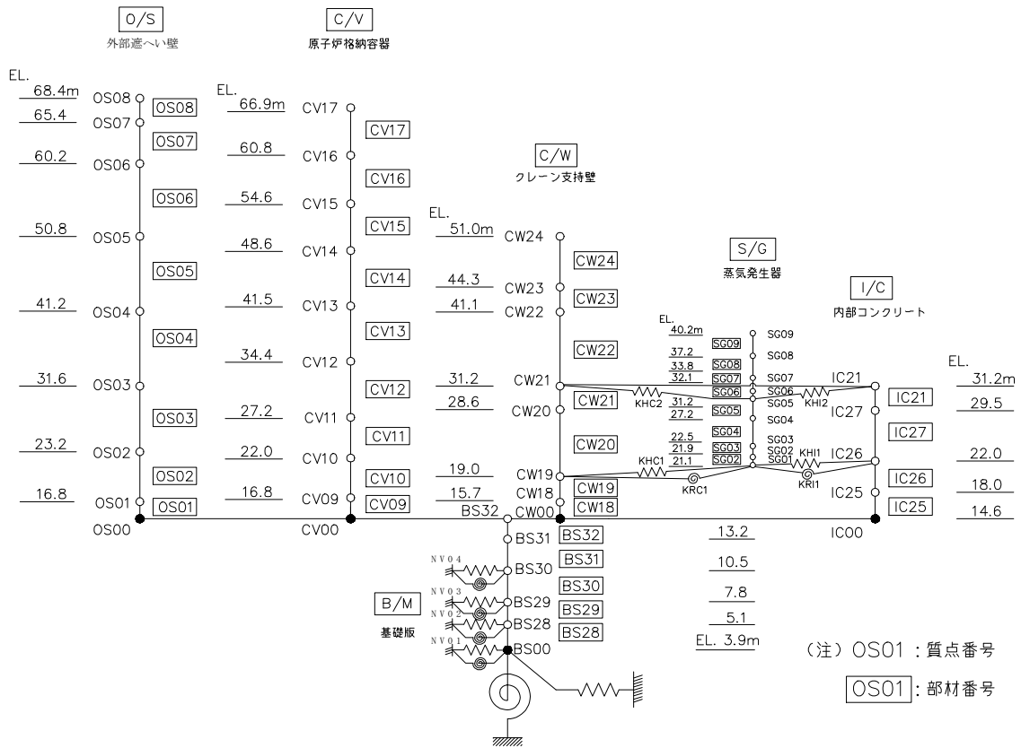
図 2 - 1 原子炉建屋の解析モデル (水平)
