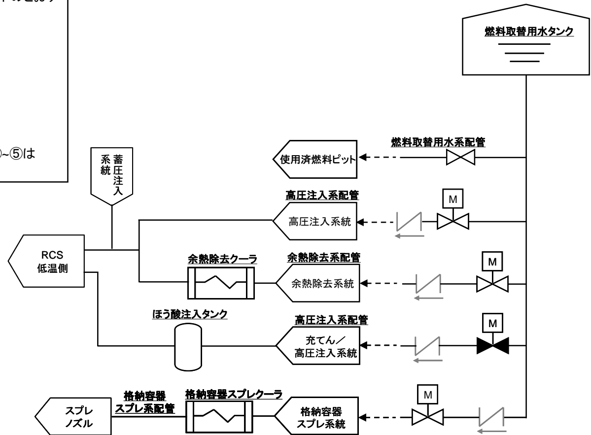
各影響緩和機能の系統図(地震:SFP燃料損傷)
