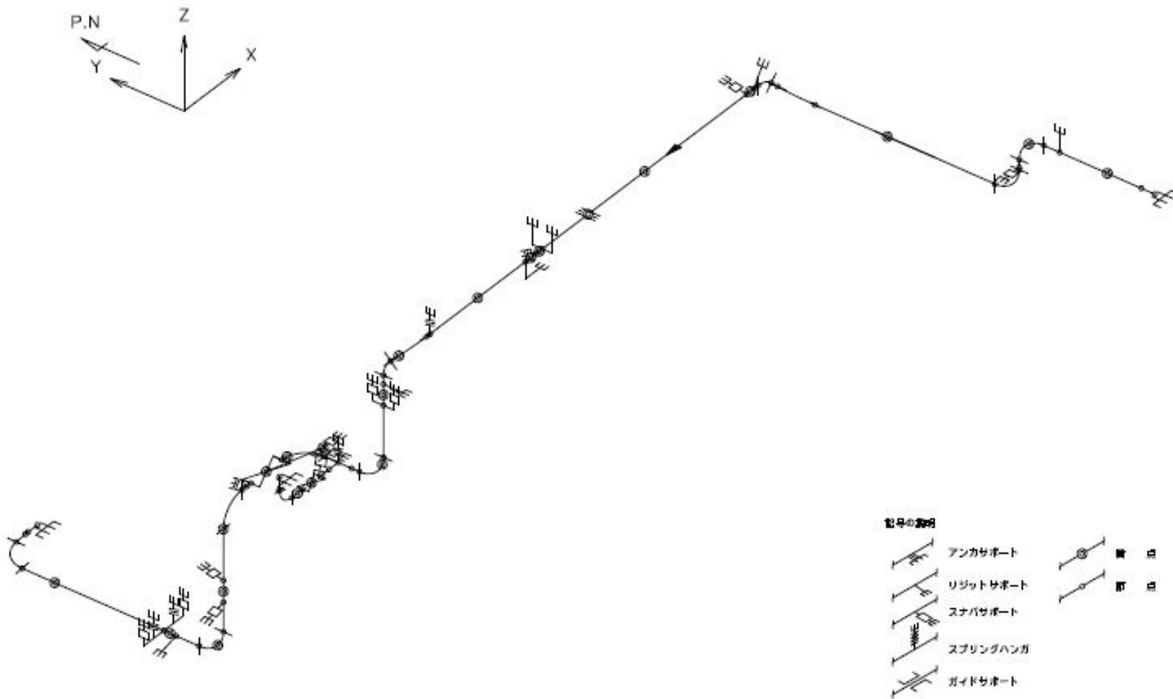
図 3 - 6 地震応答解析モデル（配管系の例）
