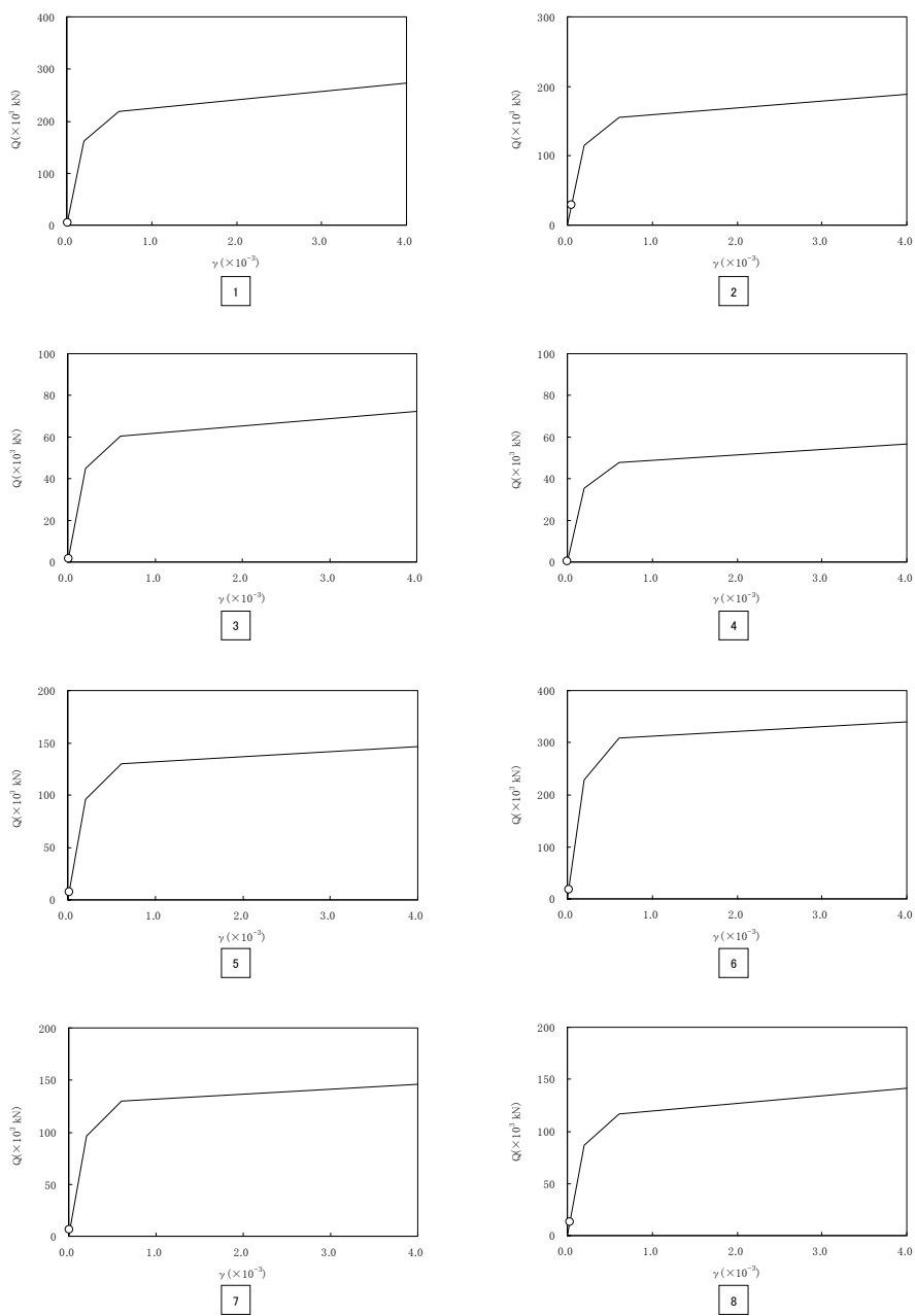
図 2-5-7 Q- \gamma 関係と最大応答値 (原子炉補助建屋 S_{S-1} EW 方向)
