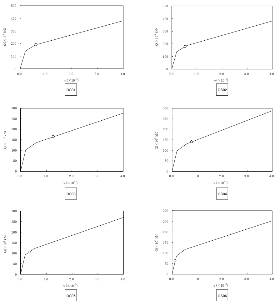
図 2-5-1 Q- \gamma 関係と最大応答値 (原子炉建屋 O/S S_{S-1} EW 方向)
