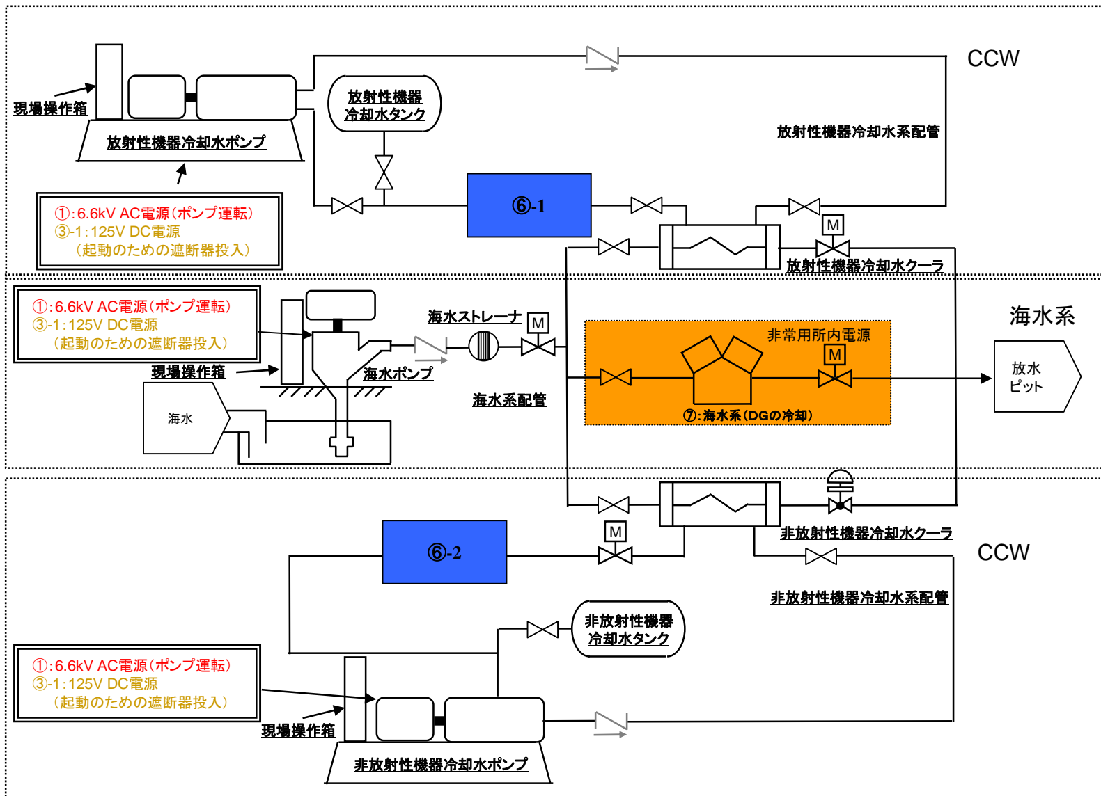
各影響緩和機能の系統図(地震:炉心損傷)
