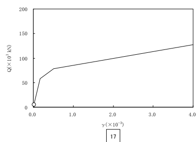
図 2-5-11 Q- \gamma 関係と最大応答値 (原子炉補助建屋 S_{S-1} NS 方向)
