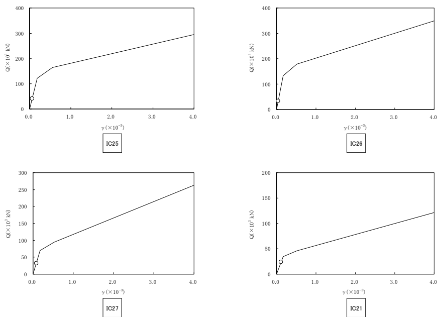
図 2-5-3 Q- \gamma 関係と最大応答値 (原子炉建屋 I/C S S-1 EW 方向)
