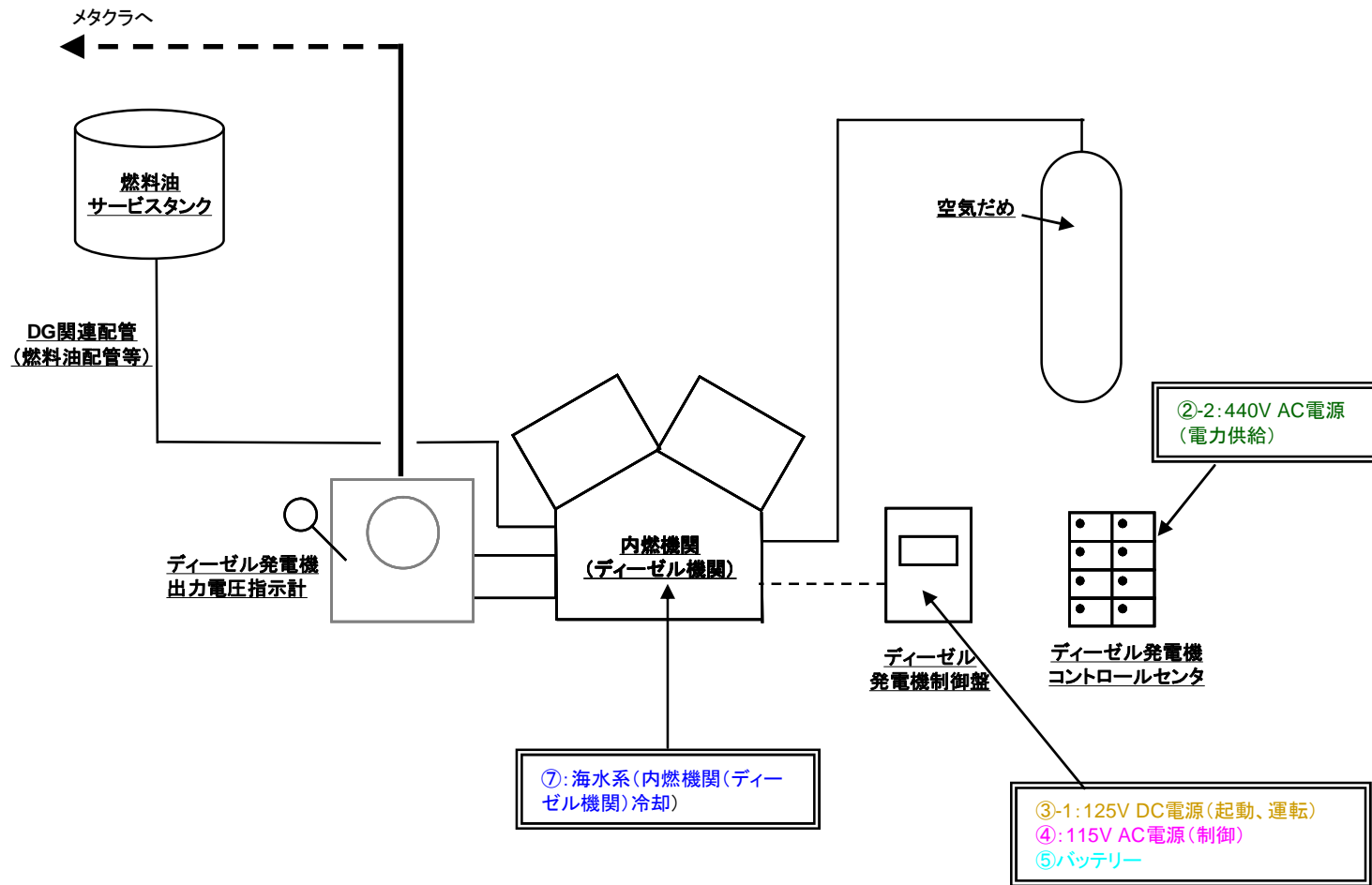
各影響緩和機能の系統図(地震:SFP燃料損傷)
