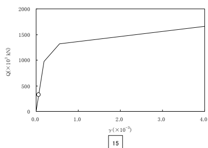
図 2-5-8 Q- \gamma 関係と最大応答値 (原子炉補助建屋 S_{S-1} EW 方向)
