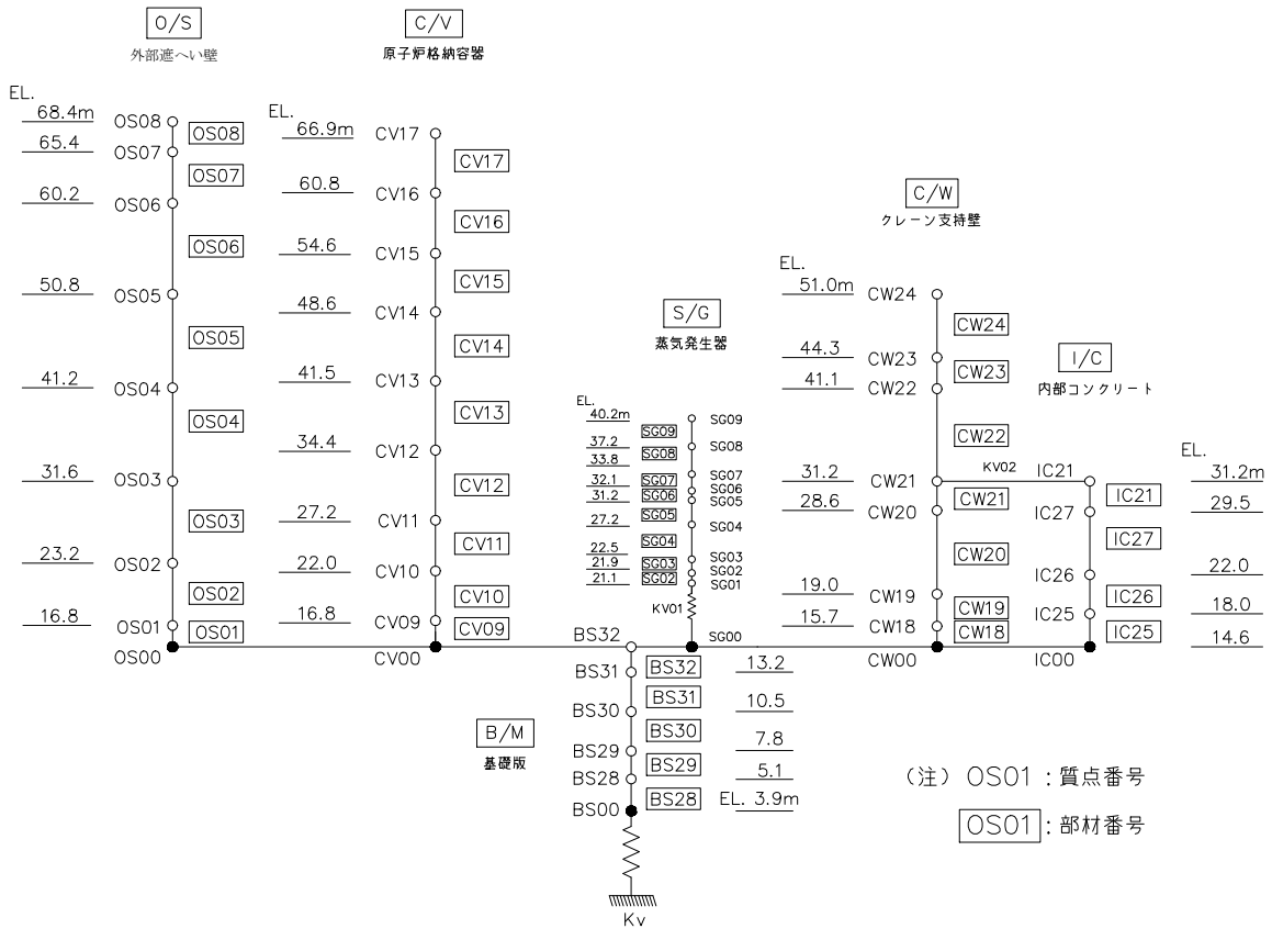
図 2 - 2 原子炉建屋の解析モデル (鉛直)
