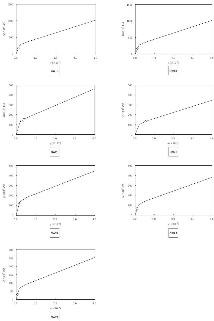
図 2-5-5 Q- \gamma 関係と最大応答値 (原子炉建屋 C/W S S-1 NS 方向)
