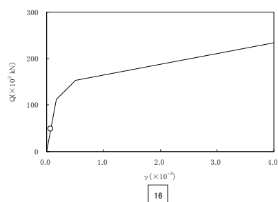
図 2-5-8 Q- \gamma 関係と最大応答値 (原子炉補助建屋 S_{S-1} EW 方向)
