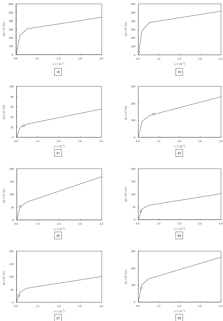
図 2 - 5 - 1 2 Q - \gamma 関係と最大応答値 (原子炉補助建屋 S_{S-1} NS 方向)
