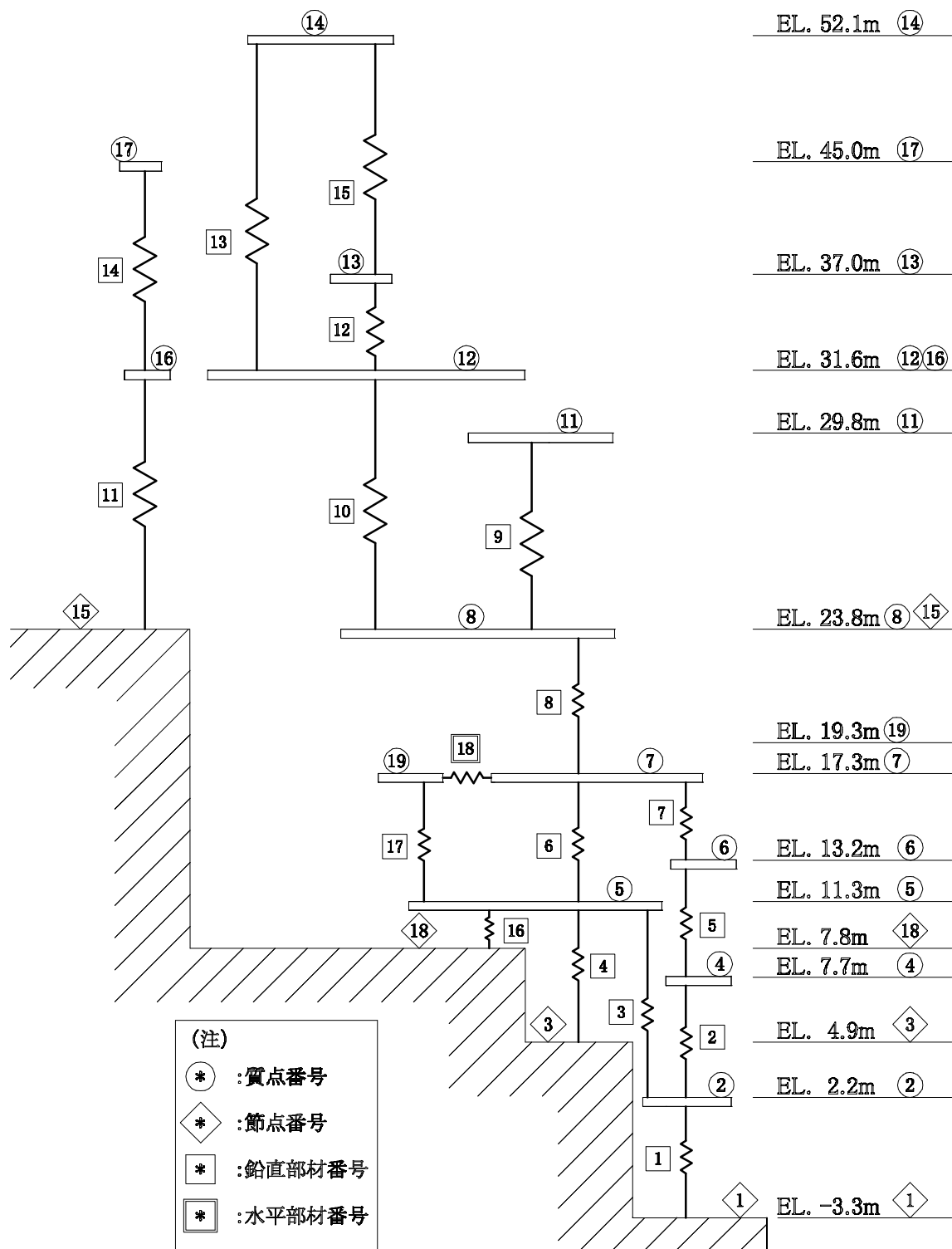
図 2 - 4 原子炉補助建屋の解析モデル(鉛直)
