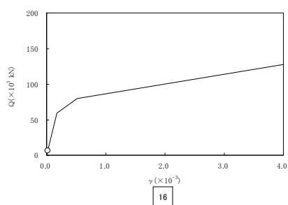
図 2-5-11 Q- \gamma 関係と最大応答値 (原子炉補助建屋 S_{S-1} NS 方向)
