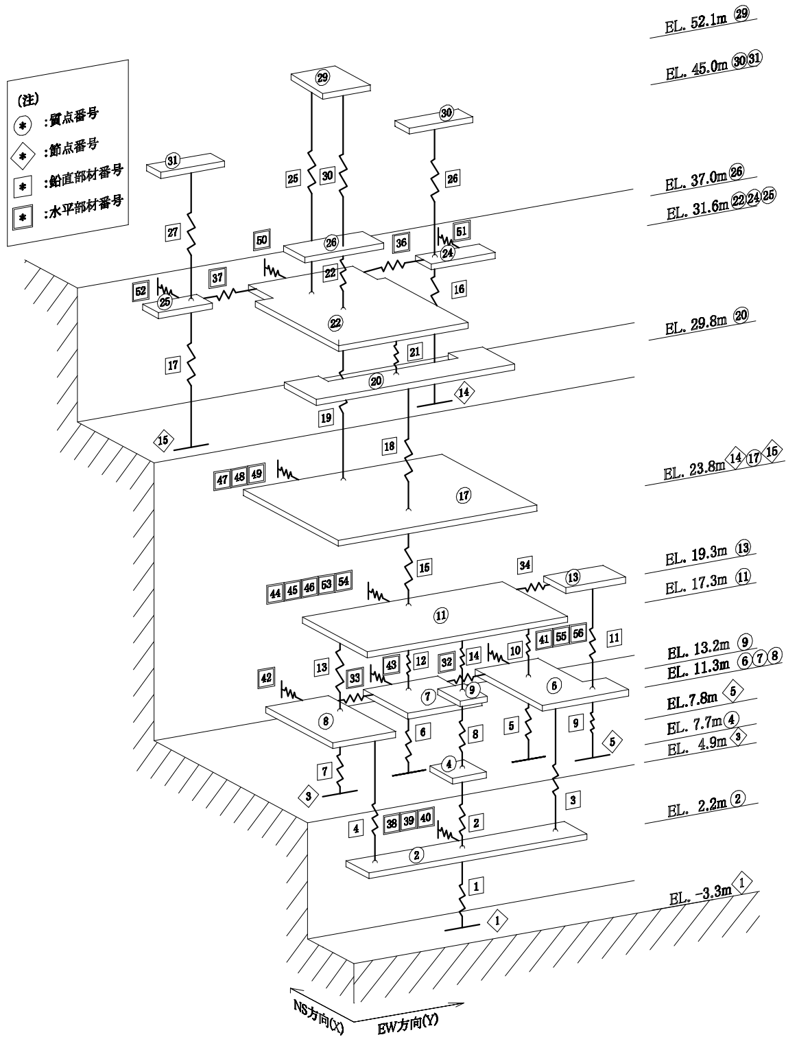
図 2 - 3 原子炉補助建屋の解析モデル(水平)
