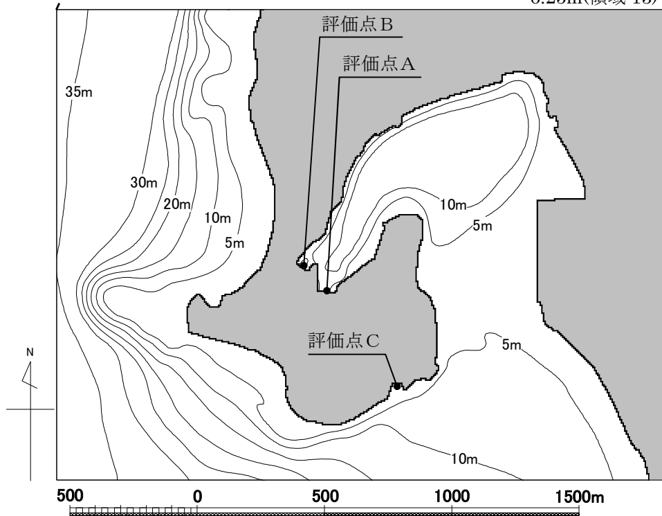
[詳細格子分割の数値計算モデル]
