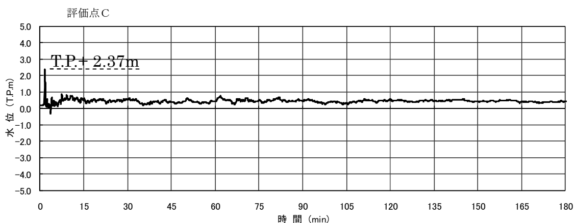
第 3-8 図 代表地点位置における水位の時系列変化 (水位上昇側: 白木-丹生断層 [広域応力場 100°, 上縁深さ 0km])
