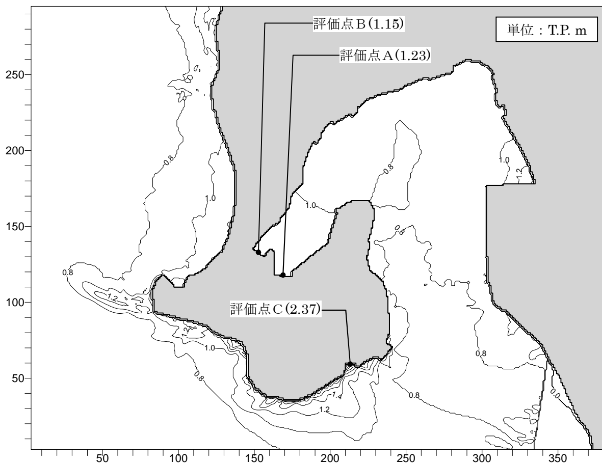
第 3-7 図 最大水位上昇量の分布 (水位上昇側: 白木-丹生断層 [広域応力場 100°, 上縁深さ 0km])
