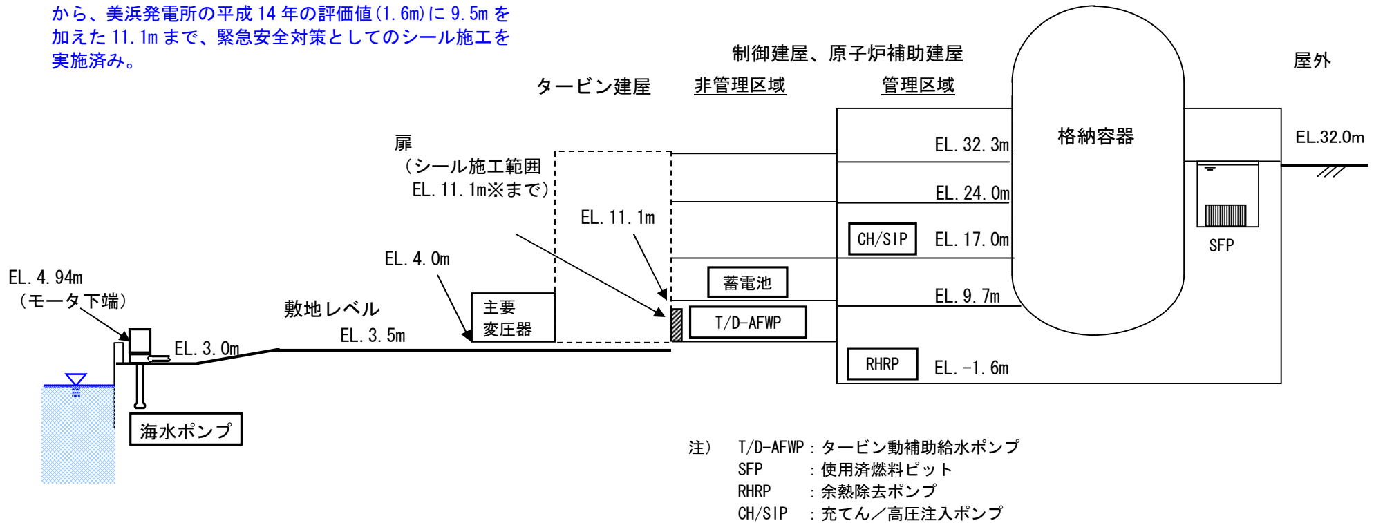
美浜 3 号機の敷地レベルと主要な機器等の配置レベル
