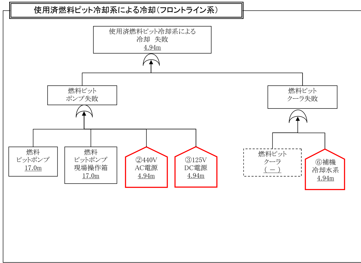
各影響緩和機能のフォールトツリー(津波:SFP燃料損傷)
