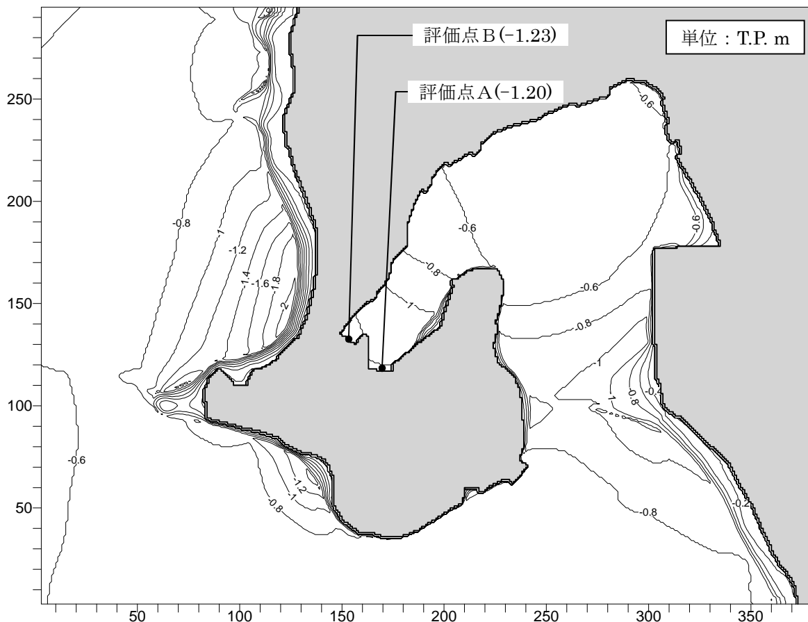
第 3-9 図 最大水位下降量の分布
