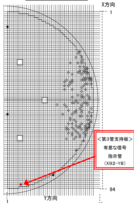
B-蒸気発生器上部より見た伝熱管位置を示す図
