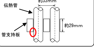
A-蒸気発生器上部より見た伝熱管位置を示す図
