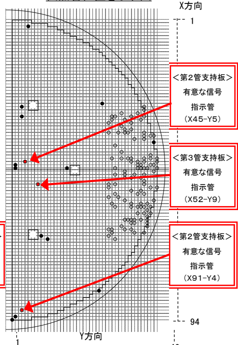
C-蒸気発生器上部より見た伝熱管位置を示す図
