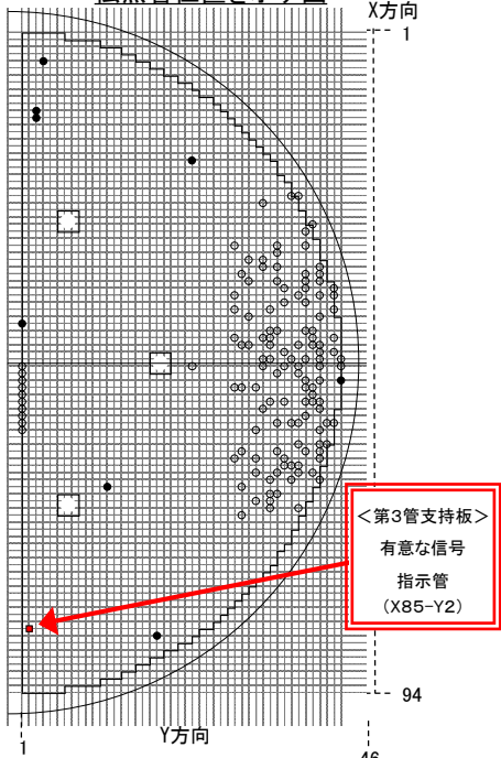
A-蒸気発生器上部より見た伝熱管位置を示す図
