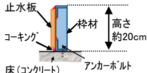
管理区域外伝播防止堰(断面図)
