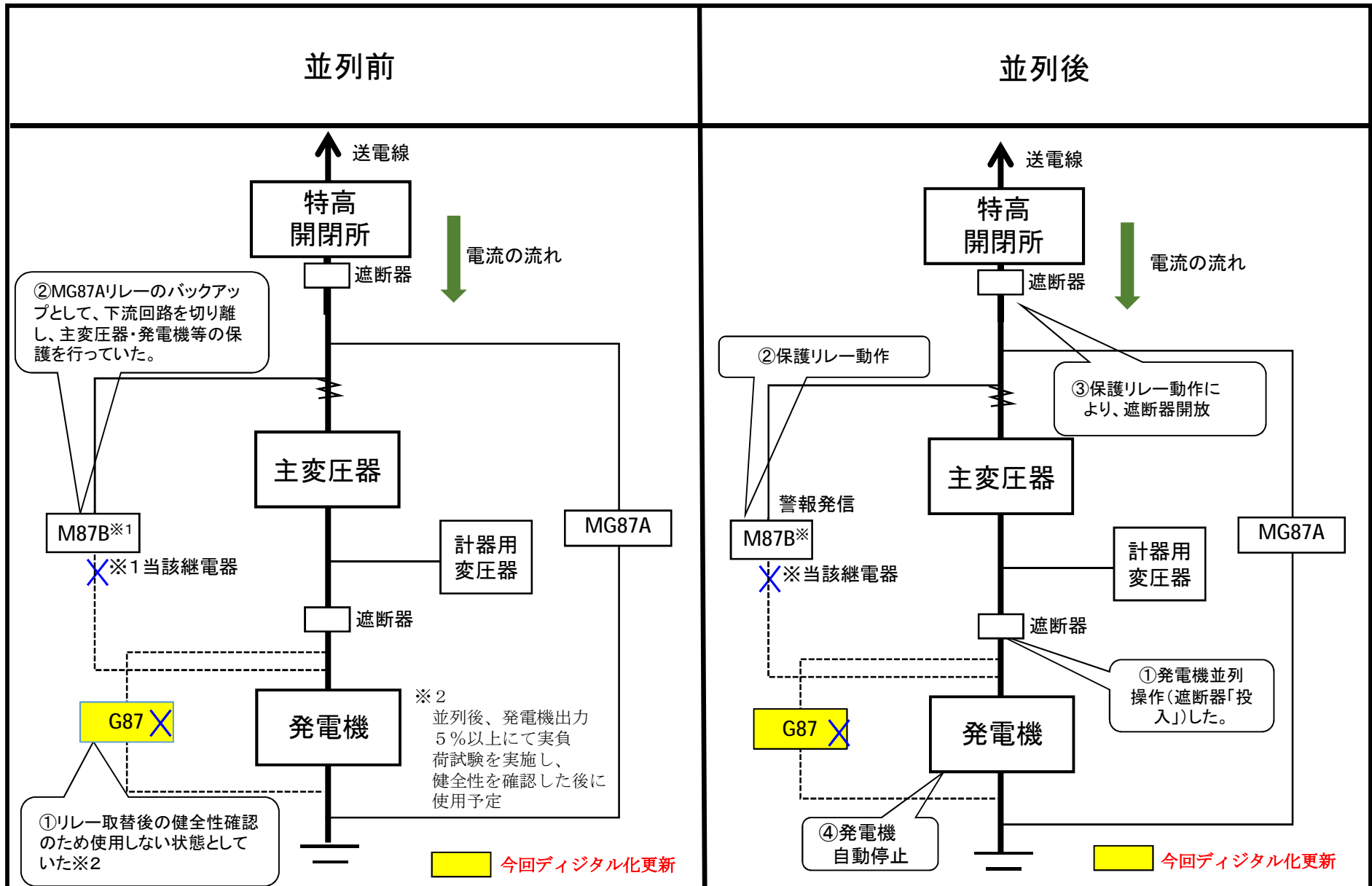
添付図1 高浜発電所4号機の原子炉自動停止について
