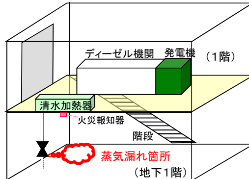
&lt;2号機A非常用ディーゼル発電機室 立面図&gt;
