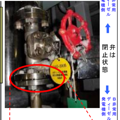
<配管フランジ部を取外した状態> (パッキングが破損)
