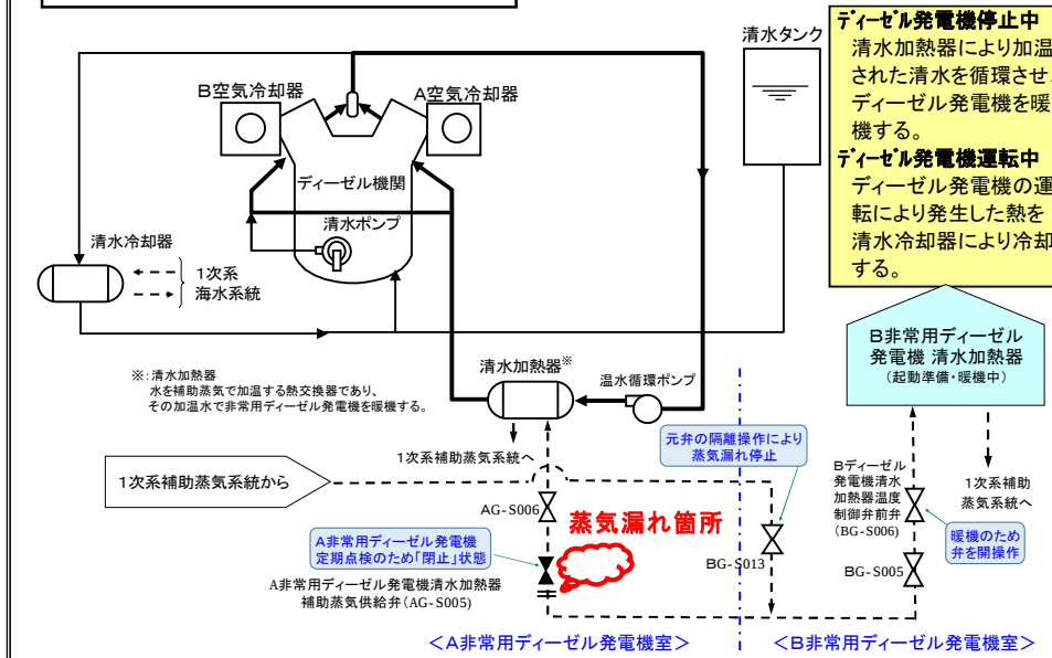
A非常用ディーゼル発電機冷却水系統概略図
