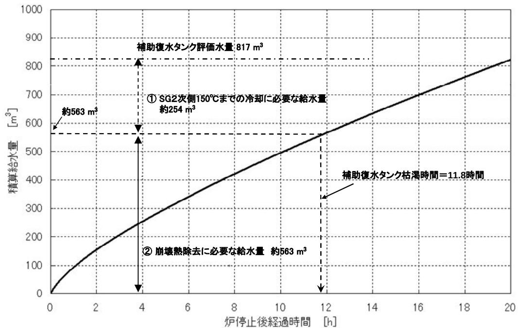
図 2 補助復水タンク水の枯渇時間評価
