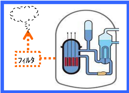
【フィルタベントの設置】 長期的避難区域の極小化 (中長期で対応)
