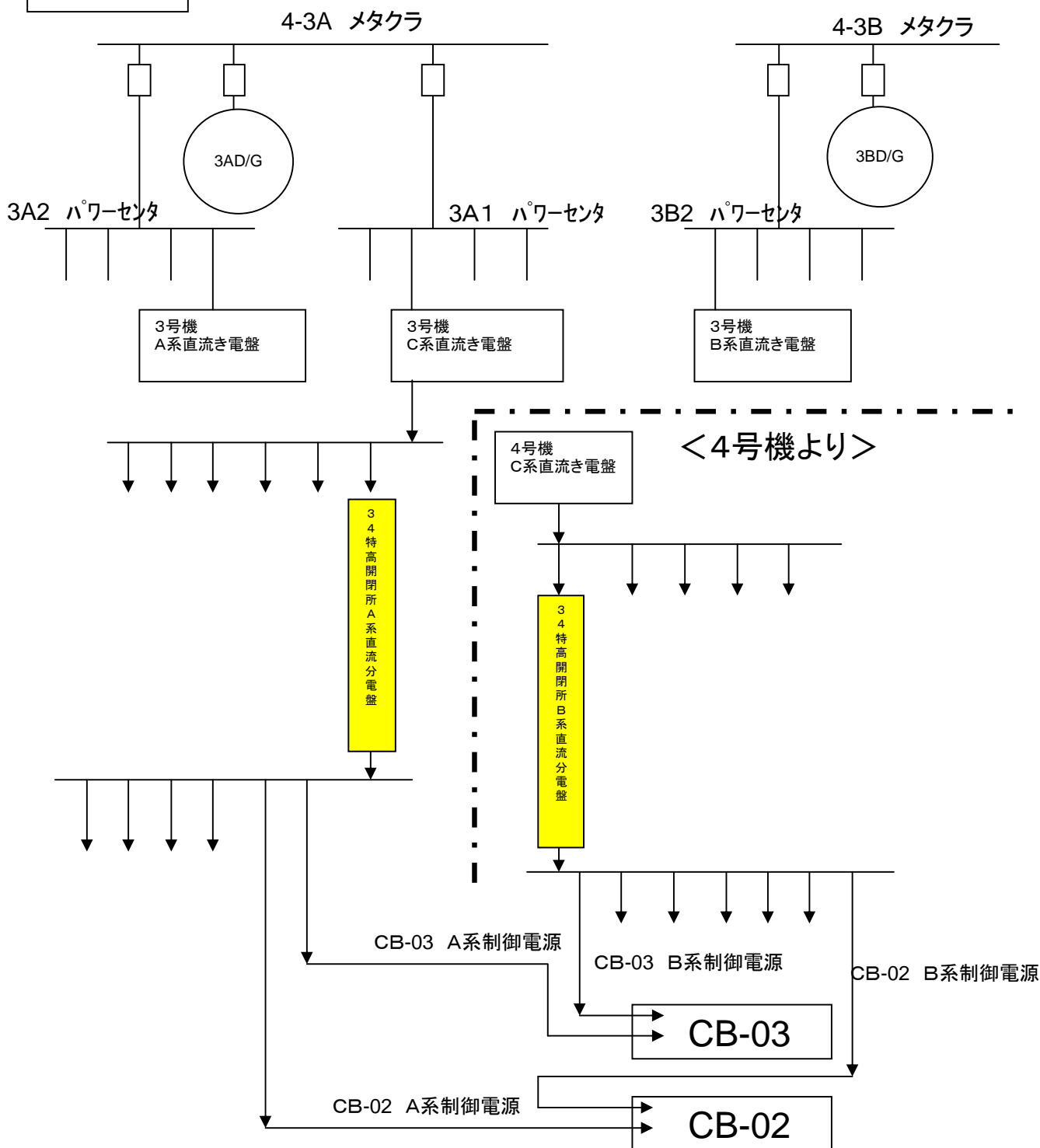
系統概要図
