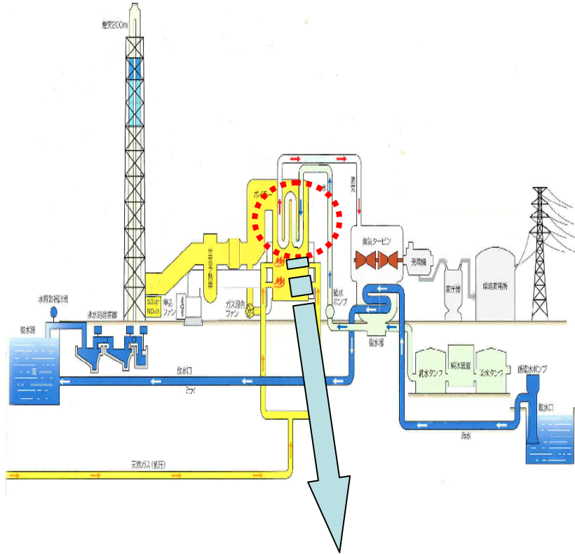
ボイラ配管の損傷状況
