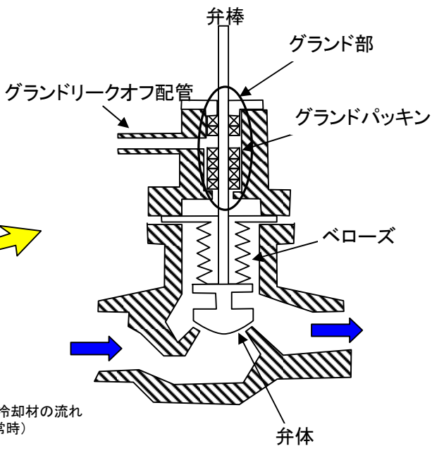
加圧器スプレ弁の拡大図
