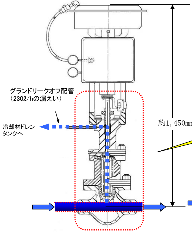
加圧器スプレ弁概要図
