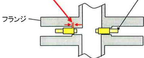
フランジ部を横から見た断面図(A-A部)
