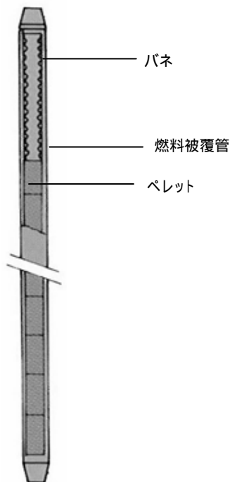
燃料棒
