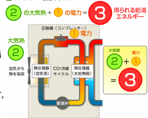
※ ヒートポンプ技術のしくみ
