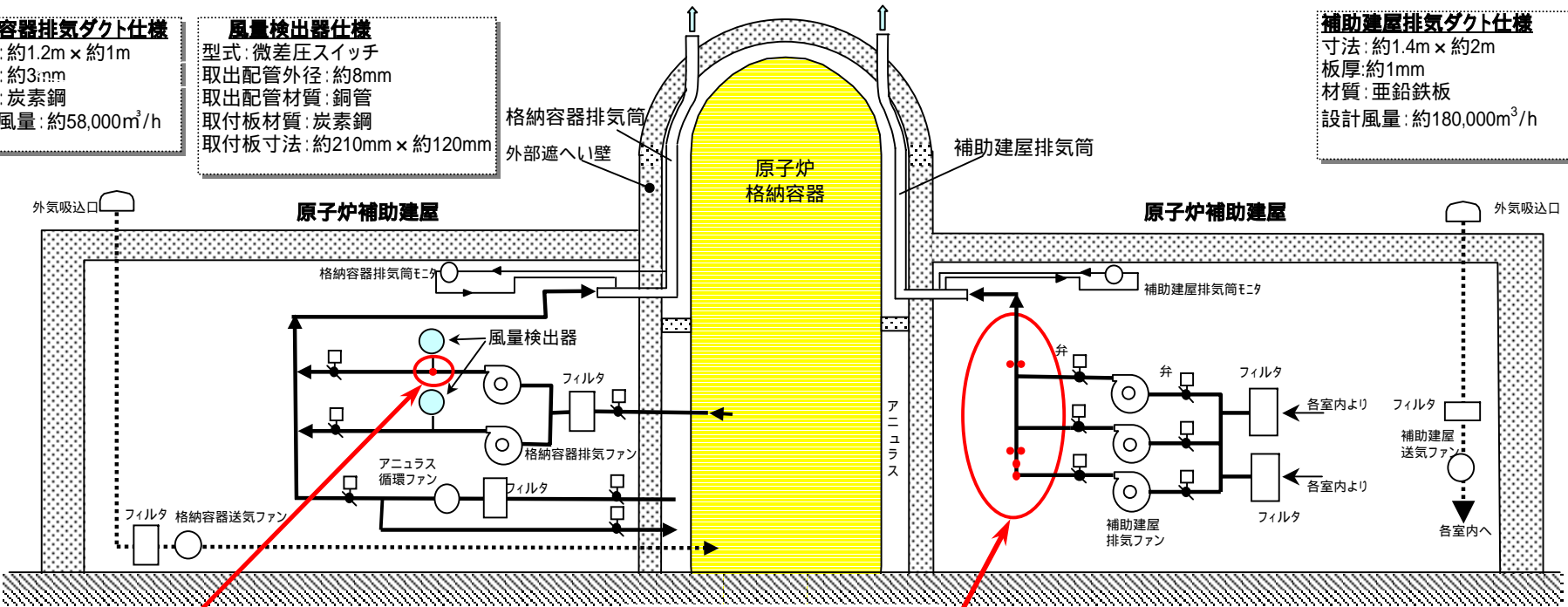
格納容器排気ダクト 風量検出器取出部 外れ箇所
