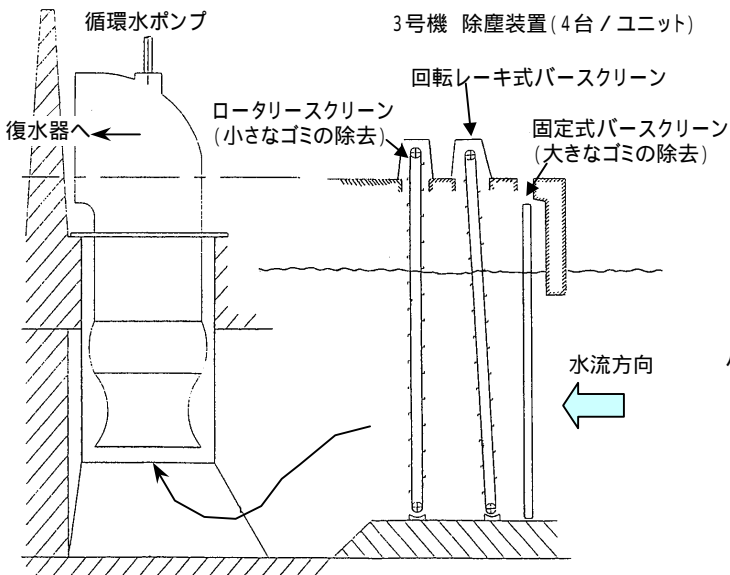
取水口機器配置図
