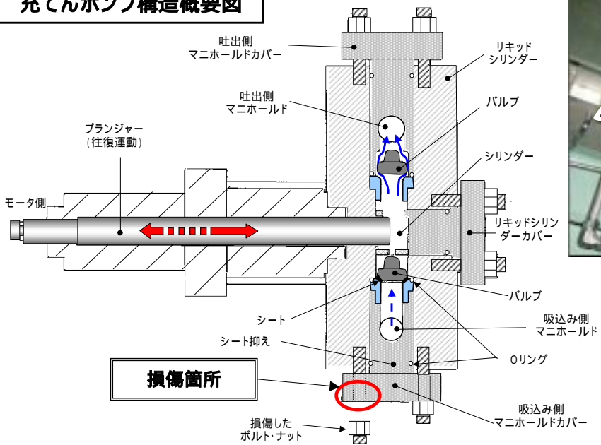
充てんポンプ構造概要図
