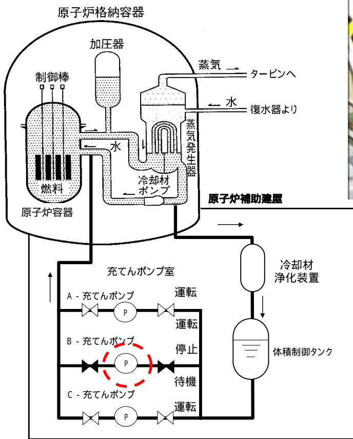
充てんポンプ構造概要図
