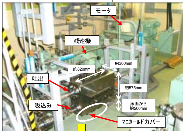
充てんポンプ外観
