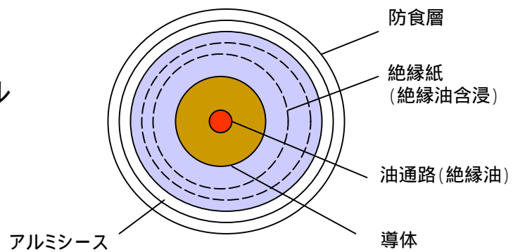
OFケーブル断面図
