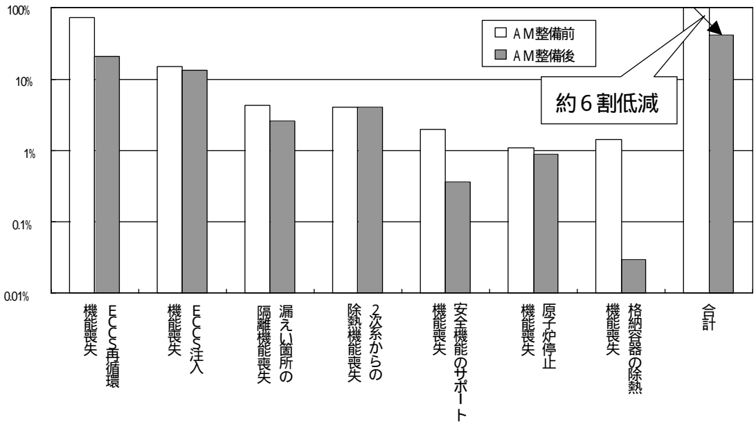
炉心の健全性に関する P S A 結果 ( 美浜発電所 3 号炉 )
