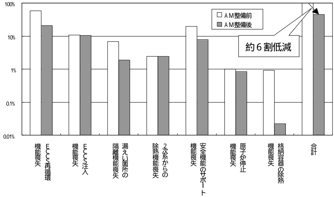
炉心の健全性に関する P S A 結果 ( 美浜発電所 1 号炉 )
