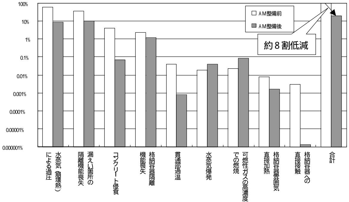
格納容器の健全性に関する P S A 結果 ( 美浜発電所 2 号炉 )
