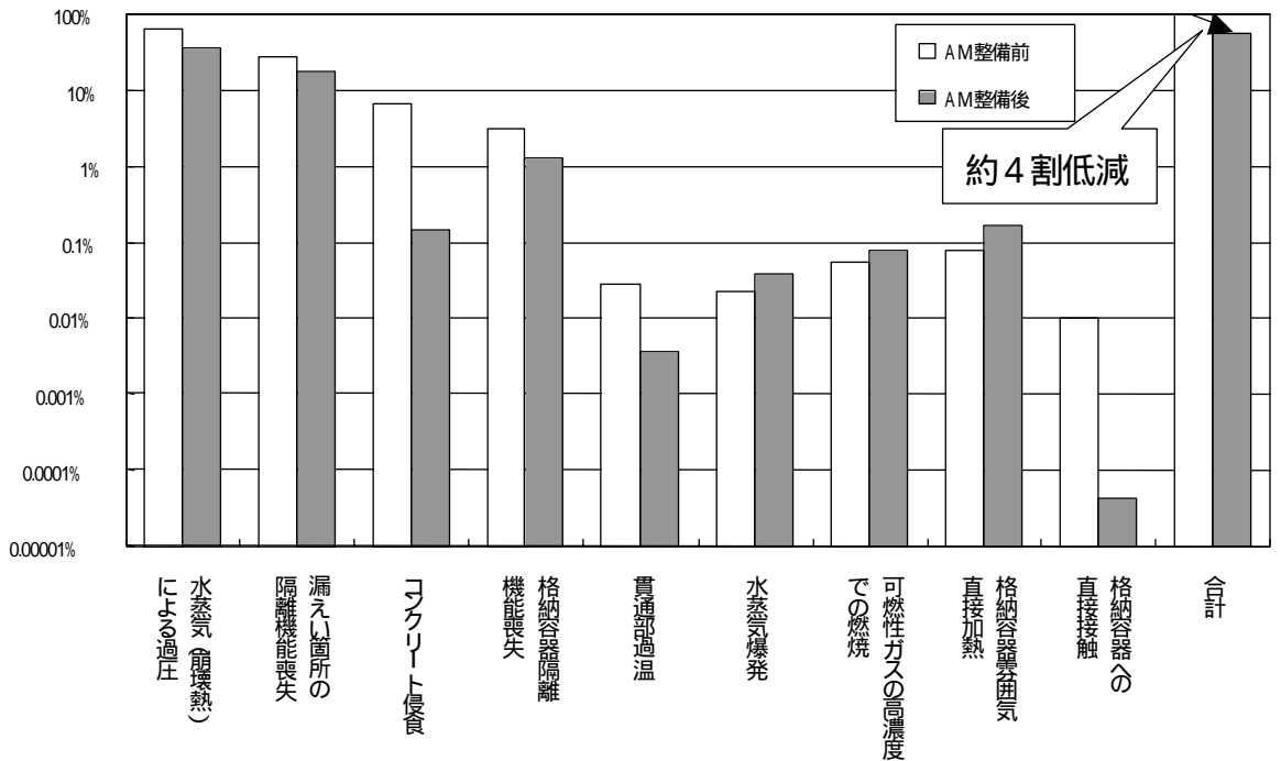
格納容器の健全性に関する P S A 結果 ( 美浜発電所 3 号炉 )
