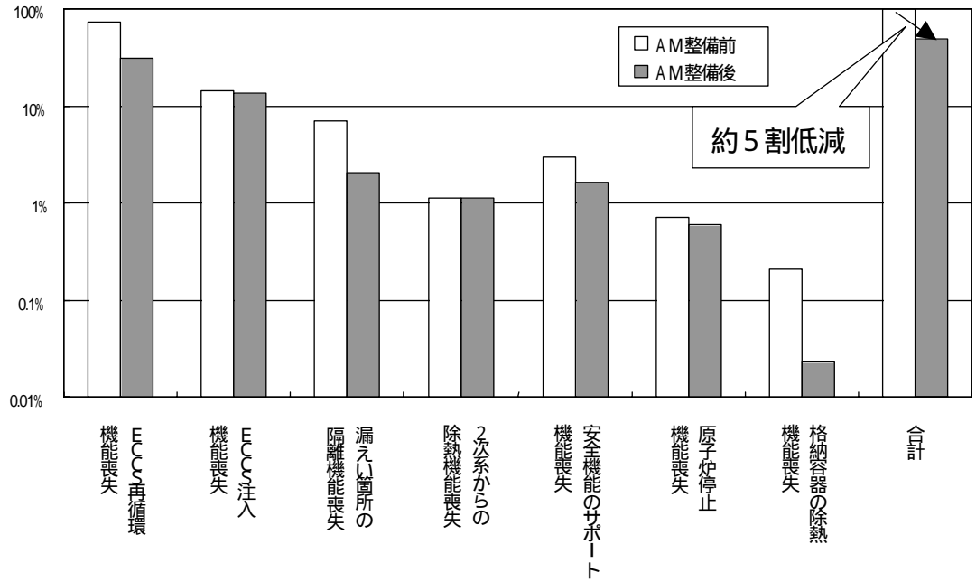
炉心の健全性に関する P S A 結果 ( 美浜発電所 2 号炉 )
