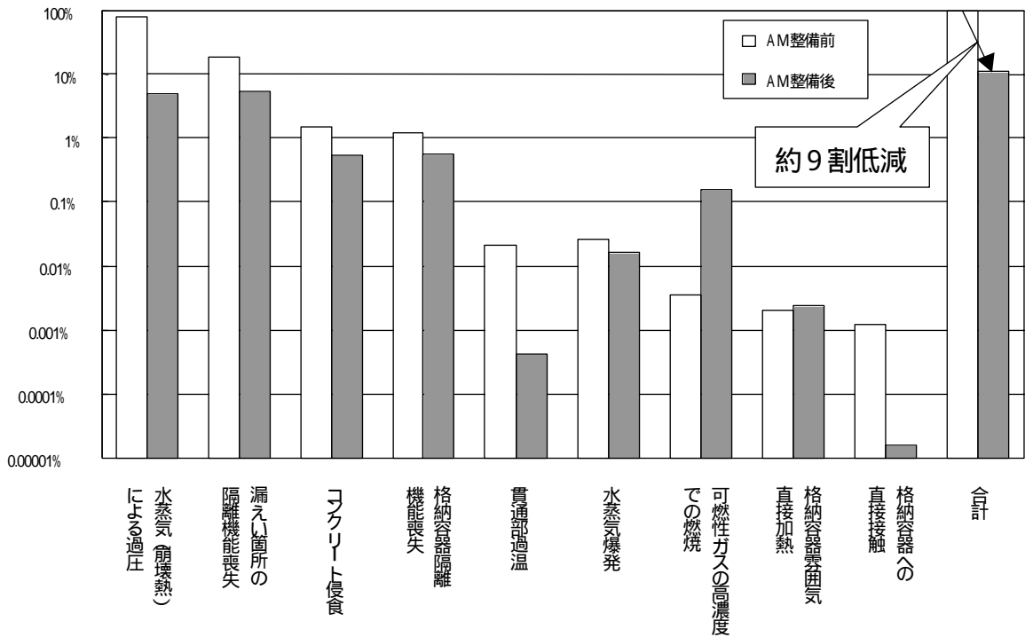
格納容器の健全性に関する P S A 結果 ( 美浜発電所 1 号炉 )
