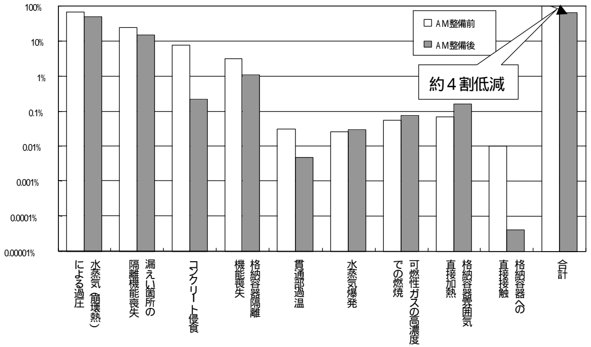
格納容器の健全性に関する P S A 結果 ( 高浜発電所 1 , 2 号炉 )
