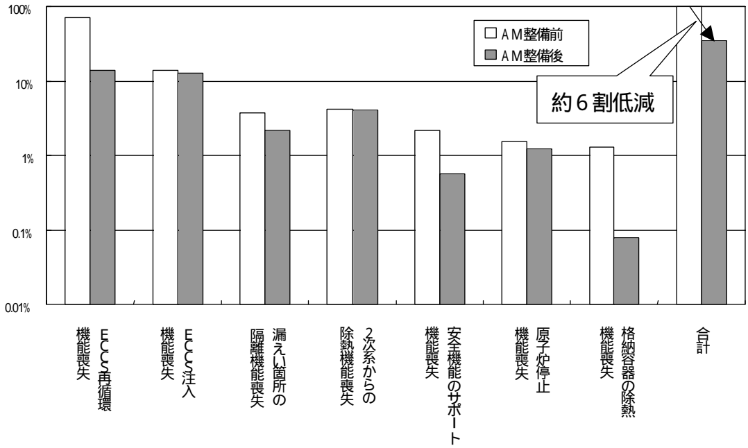
炉心の健全性に関する P S A 結果 ( 高浜発電所 1 , 2 号炉 )
