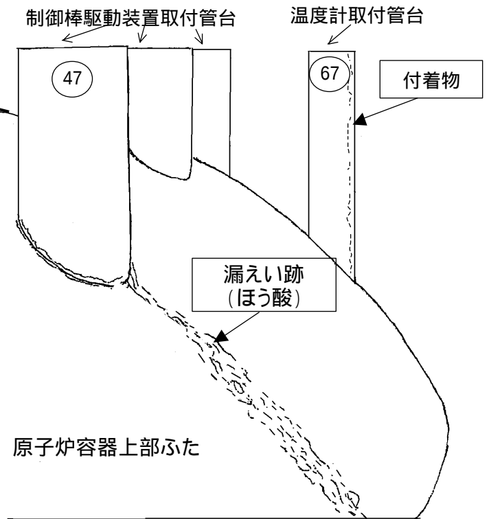
原子炉容器上部ふたの付着物状況図 (A)
