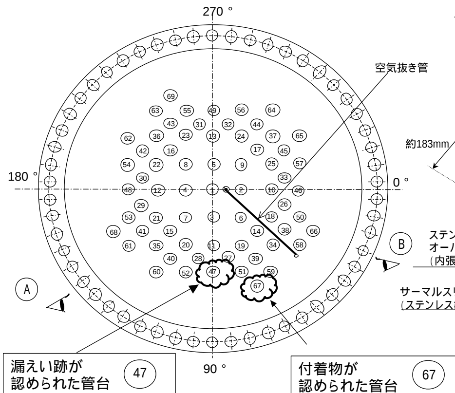
上部ふた管台配置図
