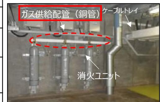
【ケーブルトレイ用消火設備】
